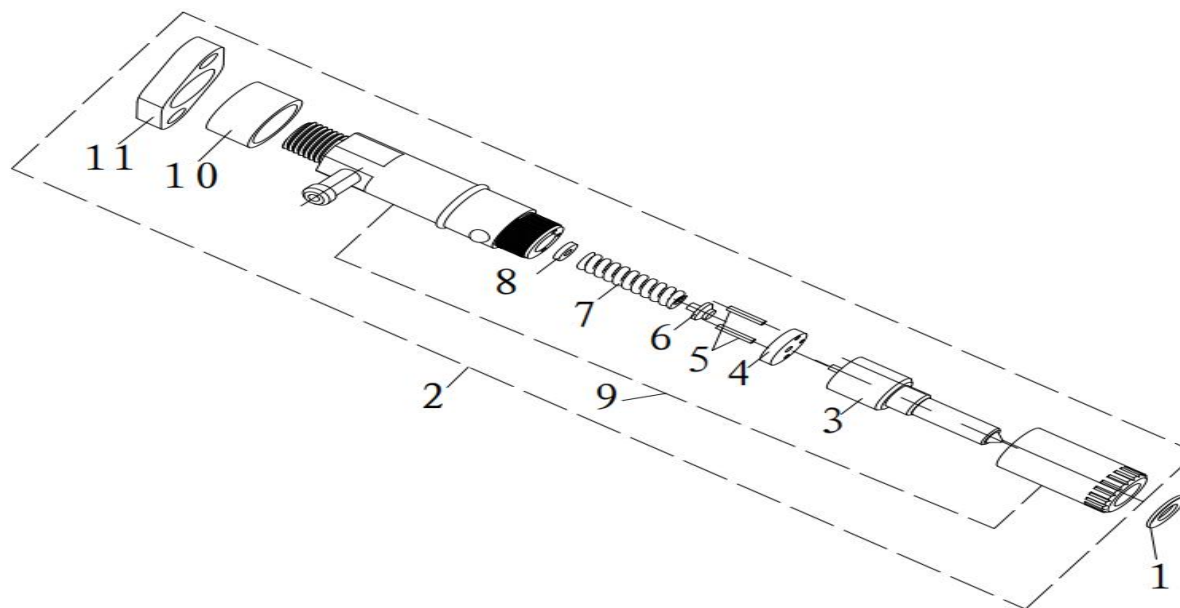
FIGUR E18 – BRÄNSLEINSPRUTNINGSENHET
