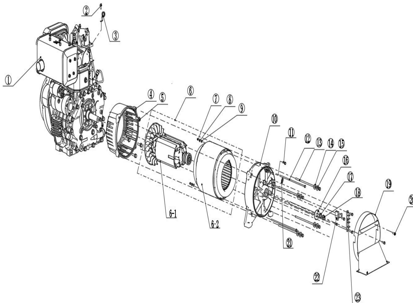
FIGUR 3 – VÄXELSTRÖMSGENERATOR
