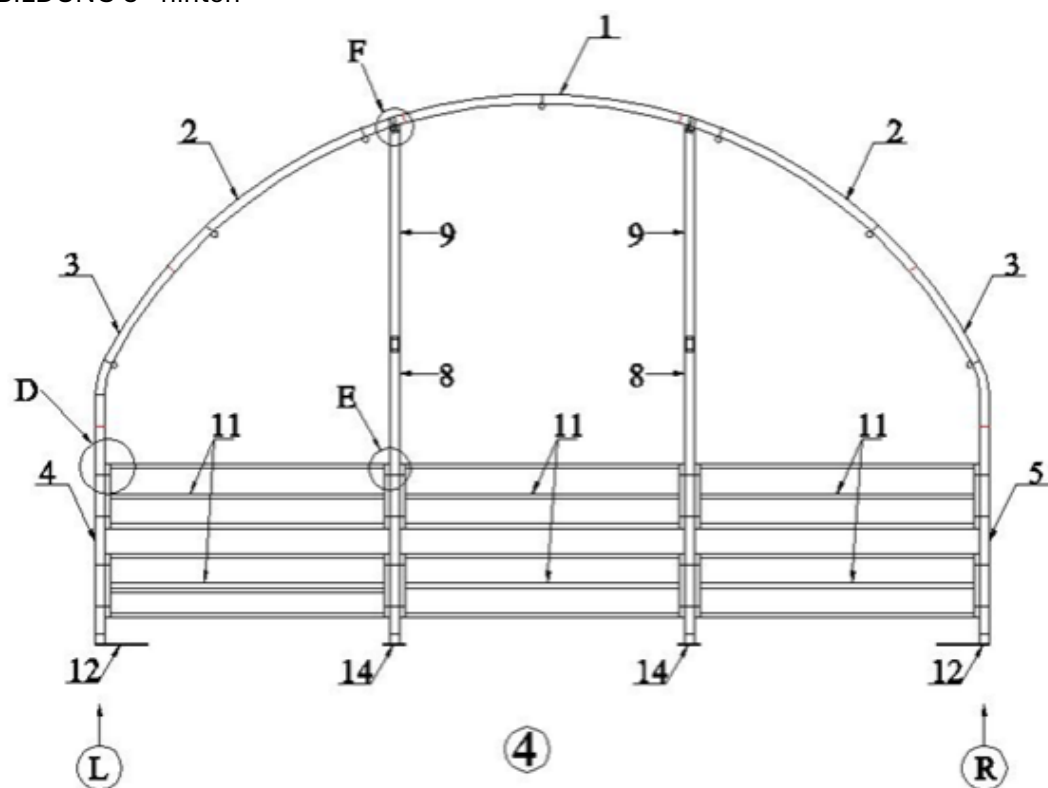
ABBILDUNG 3 - hinten
