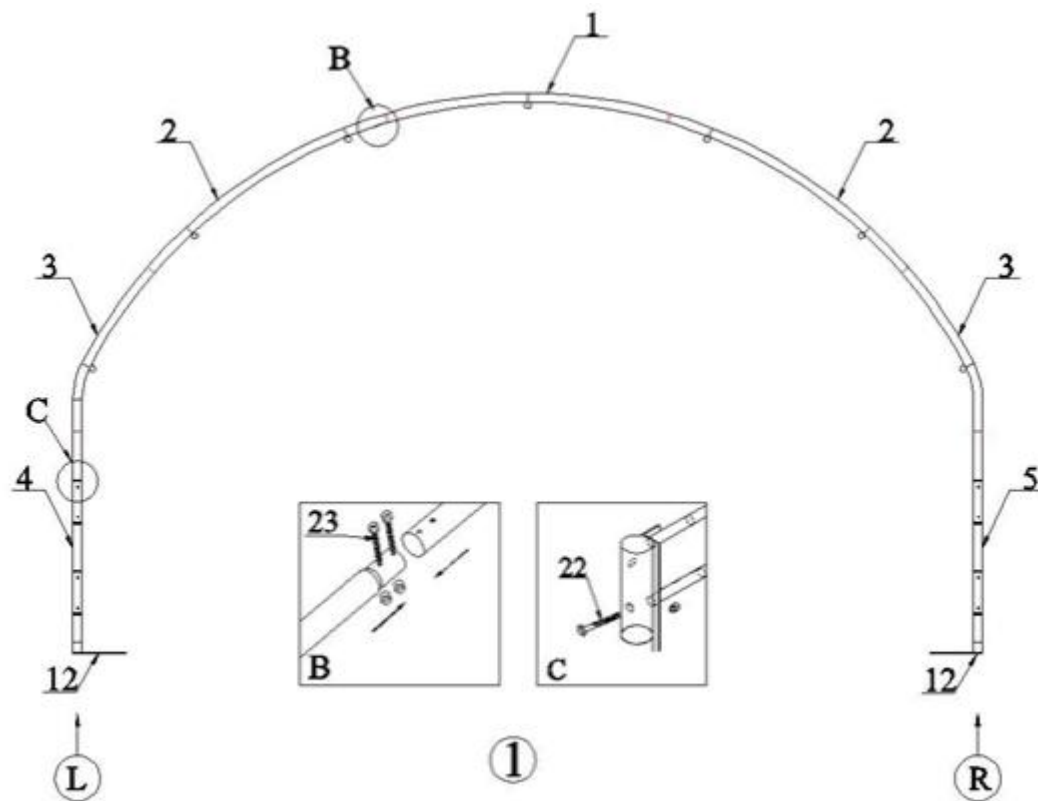
ABBILDUNG 1 - Vorderseite
