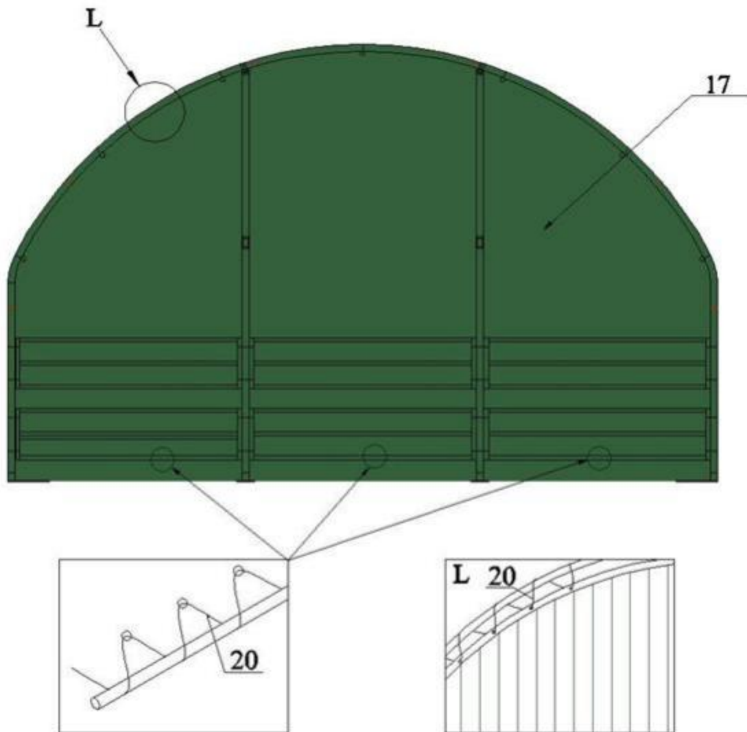
ABBILDUNG 5 – Endgiebel
