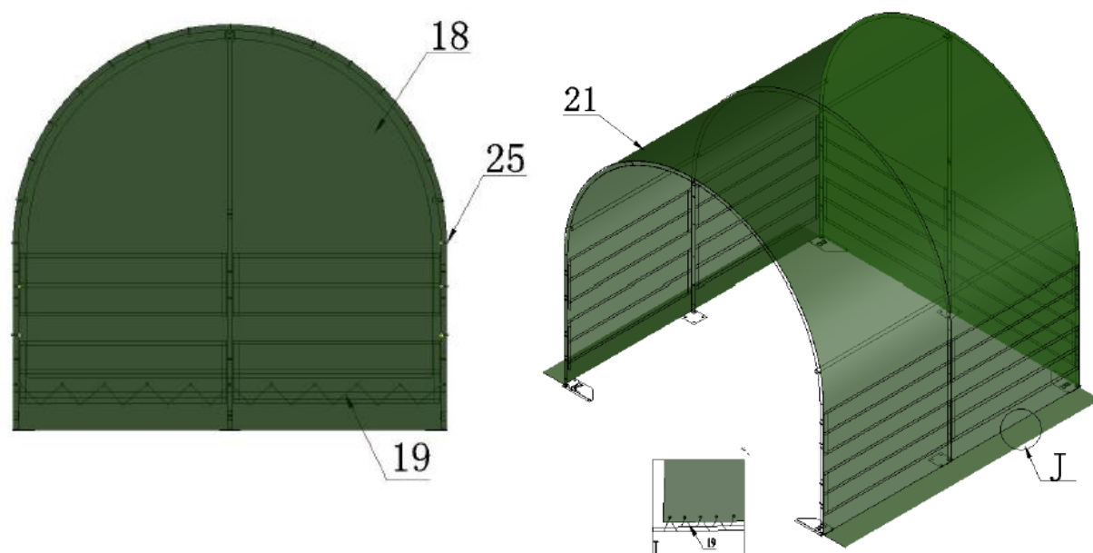
FIGUR 5 – Ändgavel och tak
