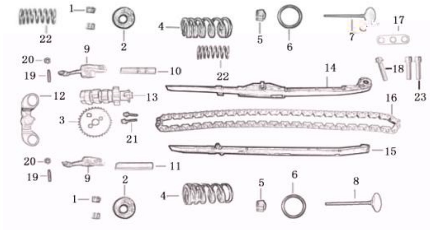
FIGUR E3 – VENTIL / VALVE
