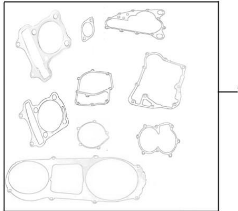
DELE TIL FIG E21 (MOTORPAKNINGSSÆT / GASKET KIT, ENGINE)
