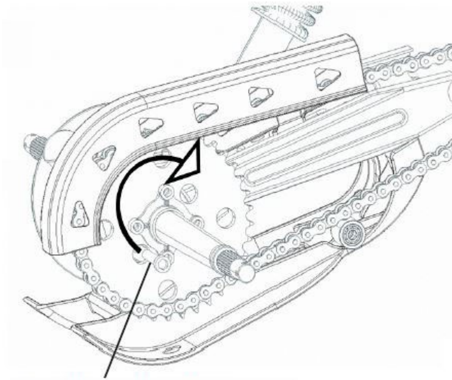
Ketteneinstellbolzen M10x60
