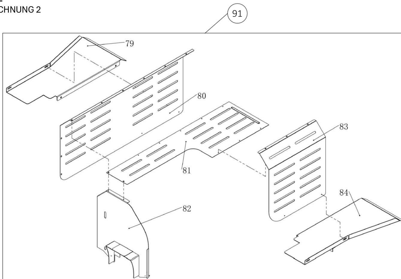
ERSATZTEILE FÜR EXPLOSIONSZEICHNUNG 2
