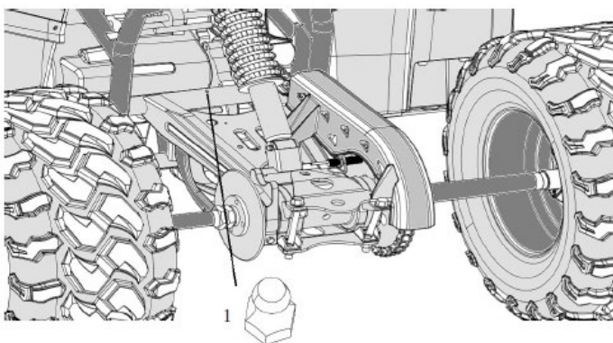
1. Smørenippel
