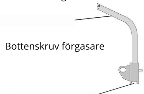
Dräneringsslang förgasare
