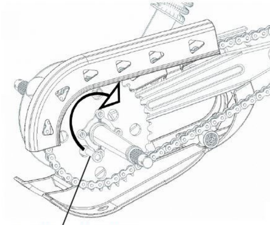
Kædejusteringsbolt M10x60
