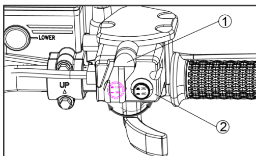
① Håndtag ② Kontakt til firehjulstræk (4WD)
