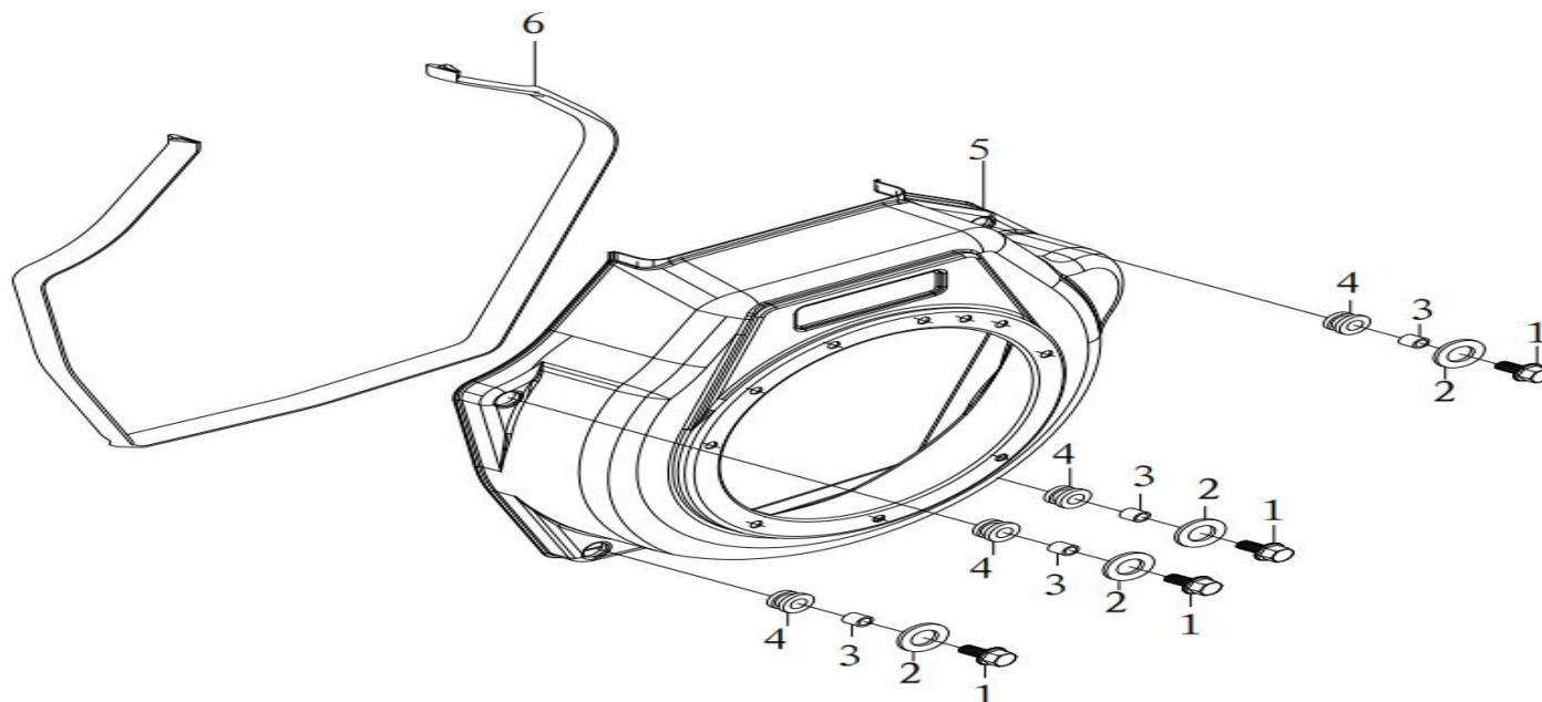
FIGUR E14 - WIND SCOOPER ASSY
