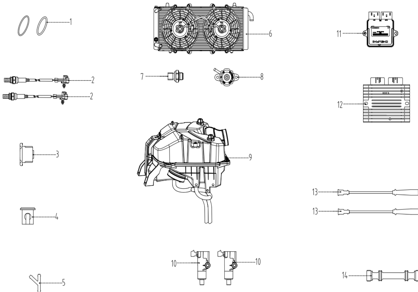
FIGUR 13 – Motor tillbehör
