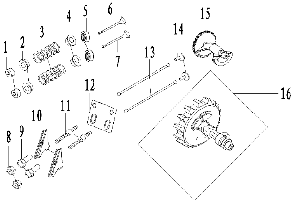
MOTOR FIGUR 5 – KAMAXEL / CAMSHAFT
