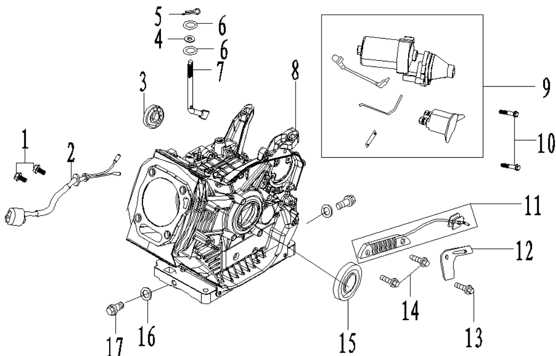
MOTOR FIGUR 2 – VEVHUS / CRANKCASE
