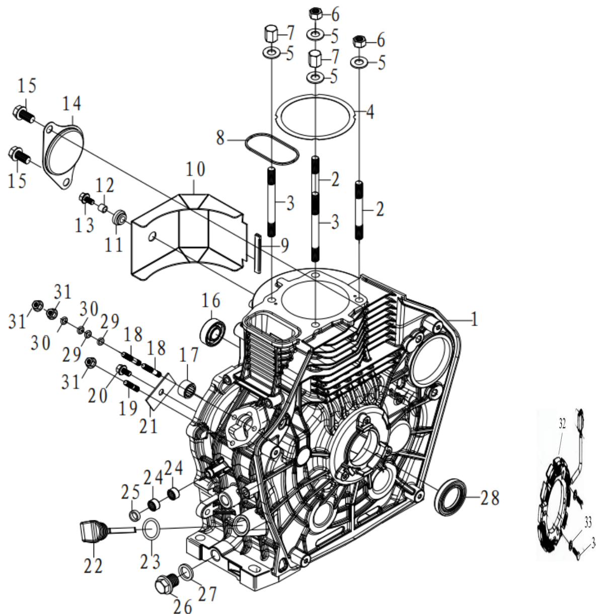
FIGUR E9 – CRANKCASE
