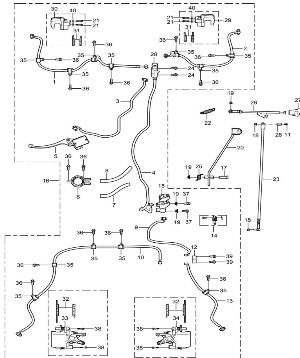
FIGUR 12 – BREMSESYSTEM, GEARSKIFTE / BRAKE SYSTEM, GEAR LEVER
