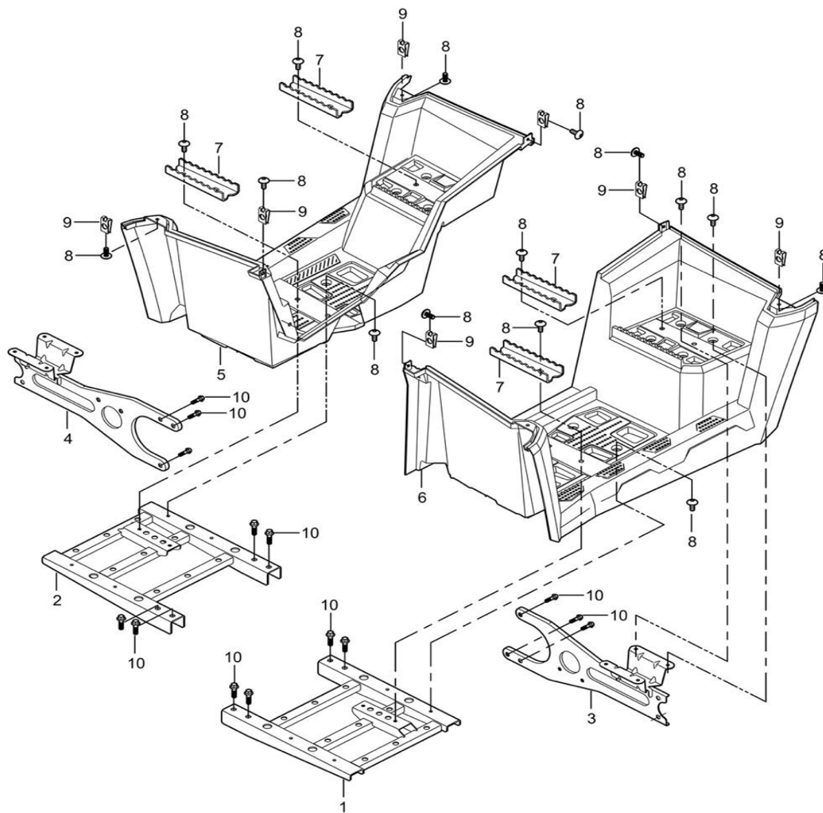
FIGUR 19 – TRINBRÆT, FODHVILER / PEDAL
