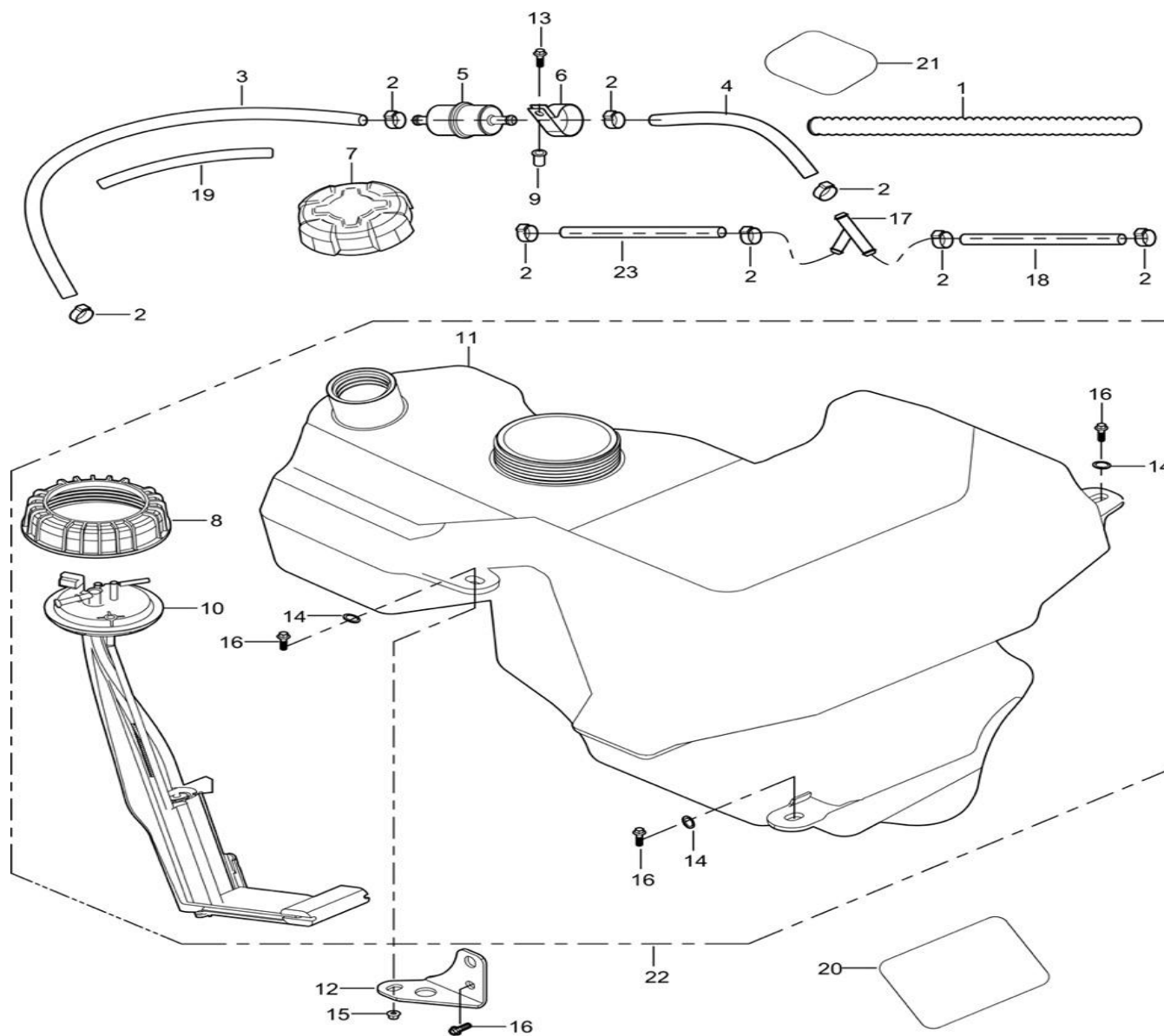
FIGUR 8 – BRÆNDSTOFSYSTEM / FUEL SYSTEM
