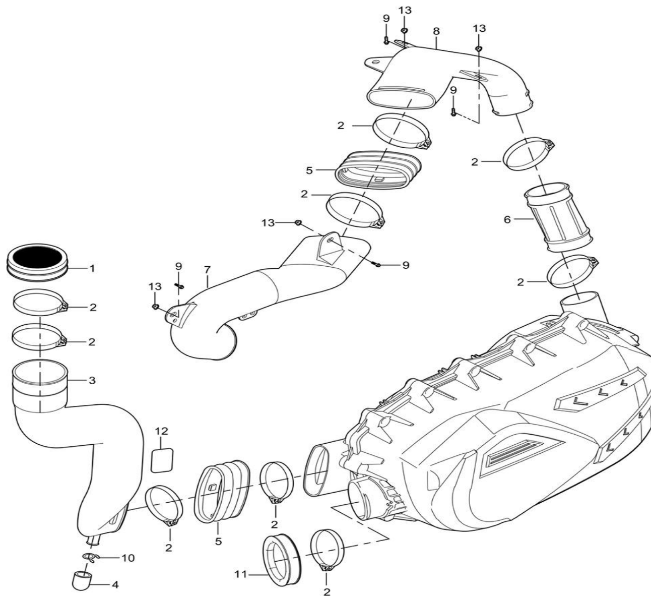
FIGUR 11 – LUFTINDTAG CVT / AIR INTAKE SYSTEM
