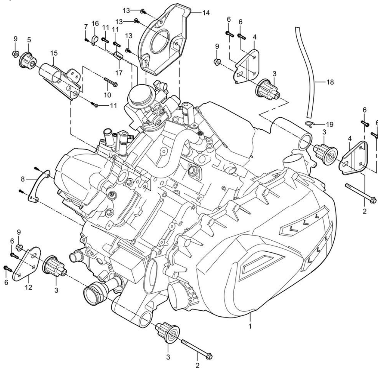
FIGUR 9 – MOTOR, OPHÆNG / ENGINE
