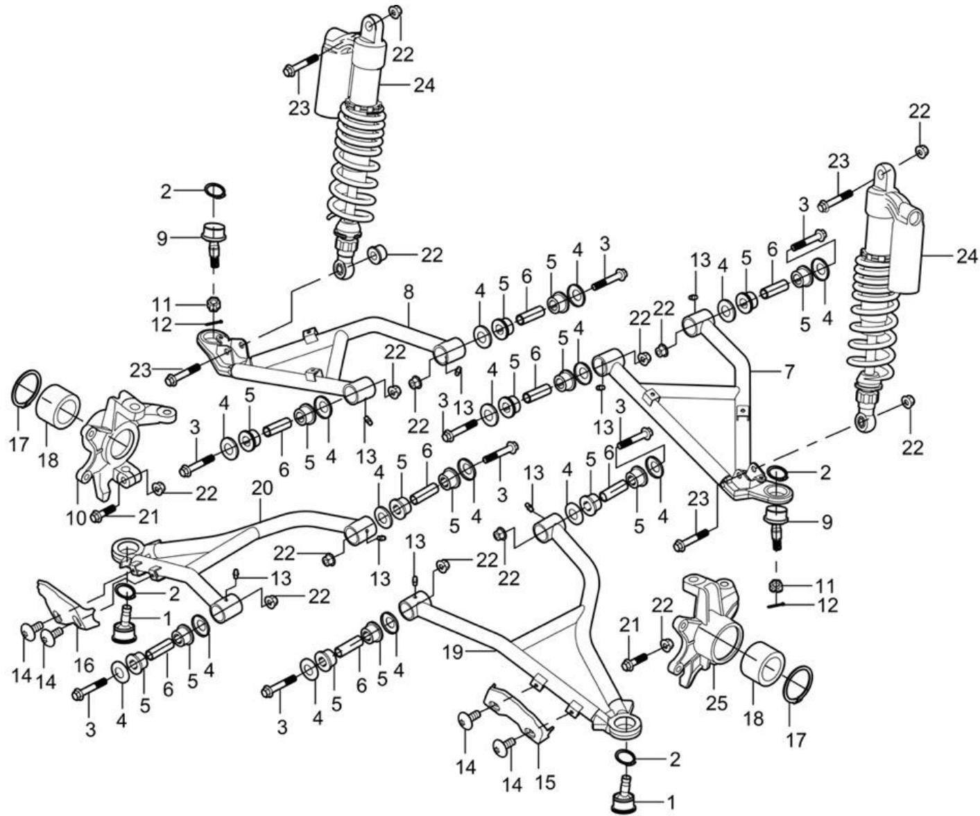
FIGUR 3 – HJULOPHÆNG, FORREST / FRONT SUSPENSION SYSTEM
