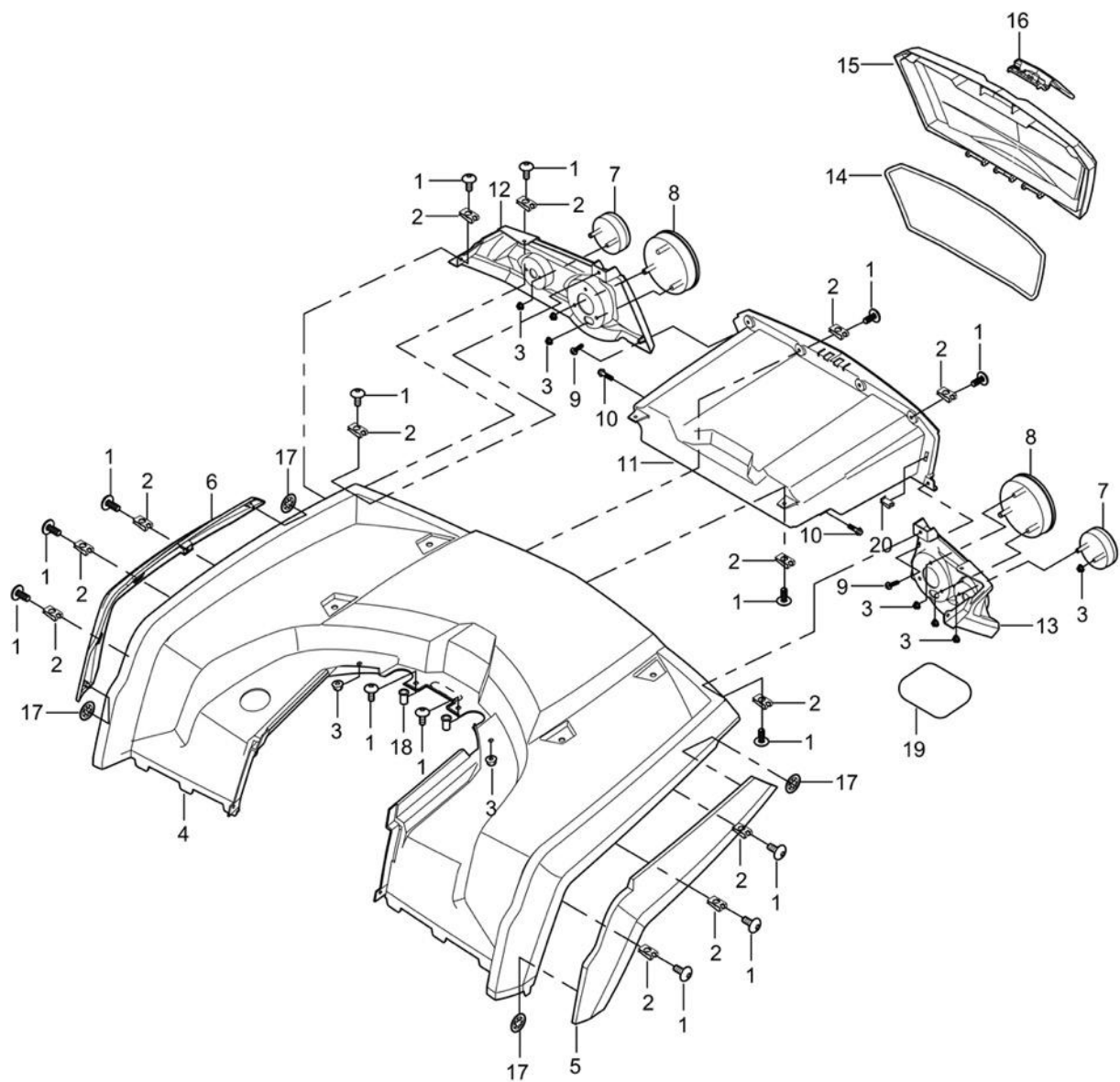
FIGUR 16 – BAGSKÆRM - TILBEHØR / REAR BODY
