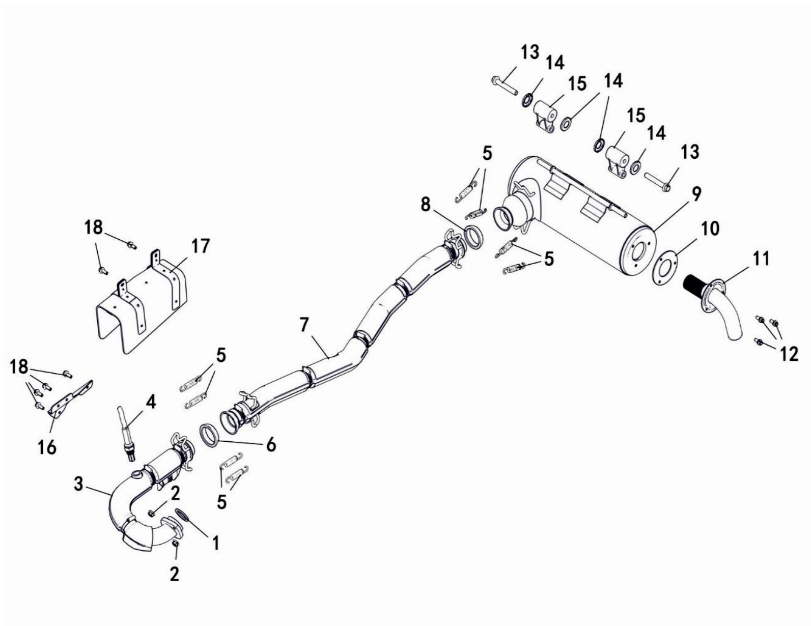
FIGUR E23 - EXHAUST T3
