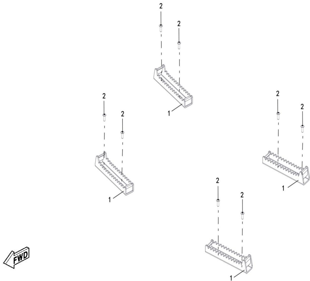
FIGUR 47 - OPTIONS (ANTISKID TEETH ASSY)
