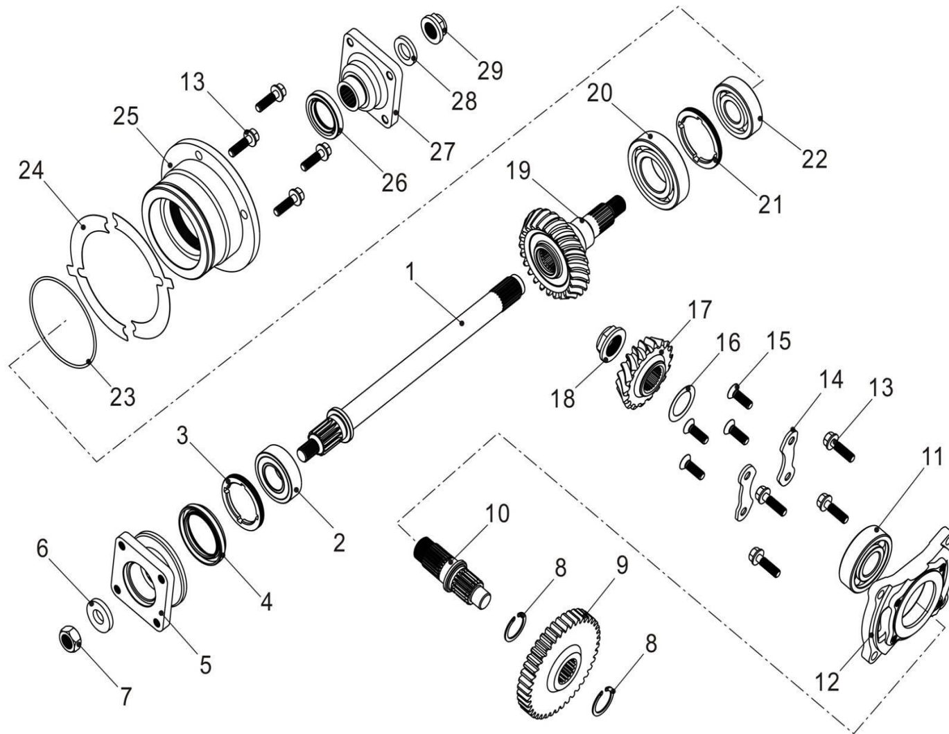
FIGUR E15 - TRANSMISSION II
