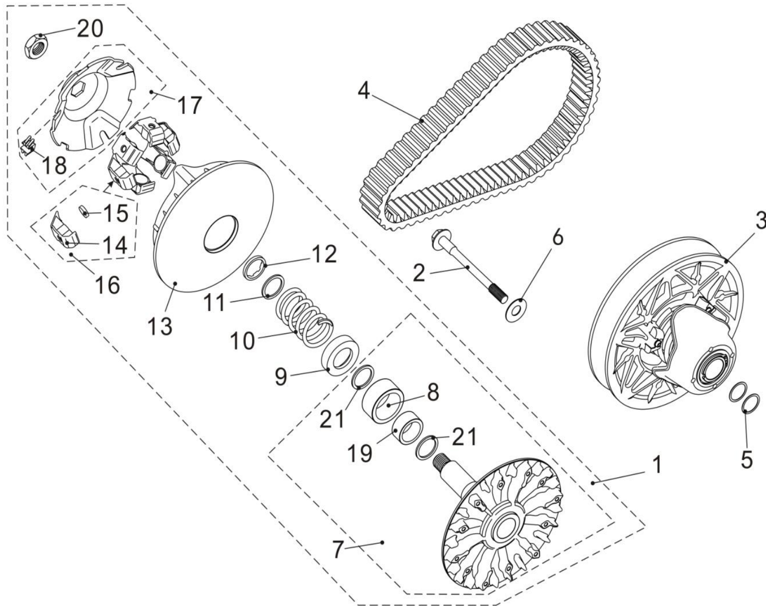
FIGUR E13 - CLUTCH
