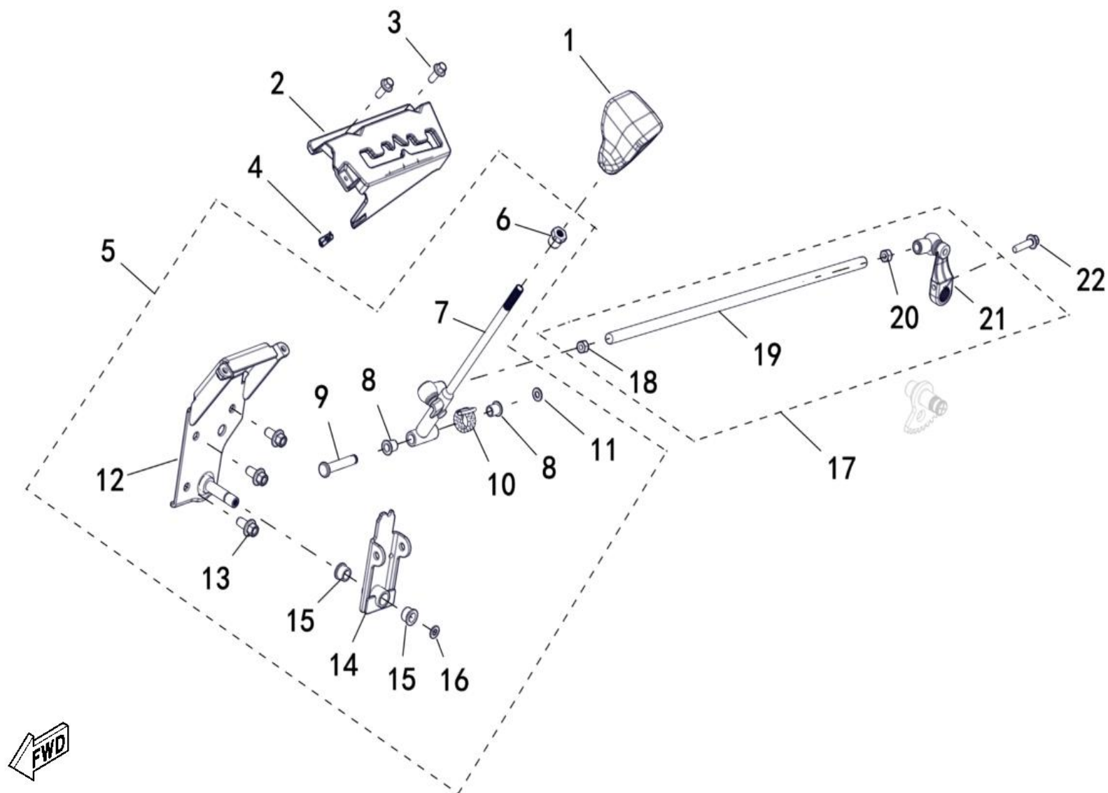
FIGUR 28 - SHIFT
