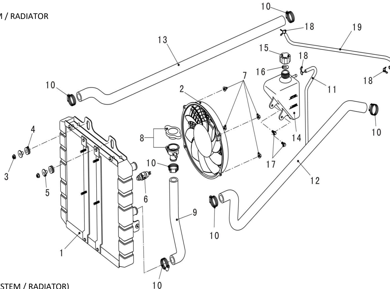
DELE TIL FIG 21 (KØLERSYSTEM / RADIATOR)
