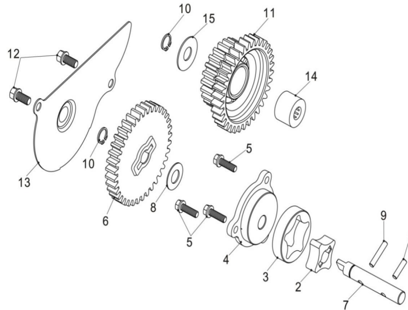
DELE TIL FIG 17 (OLIEPUMPE / OIL PUMP)
