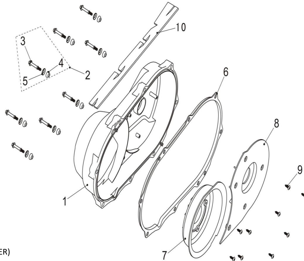
FIGUR 9 – CVT-DÆKSEL / CVT COVER
