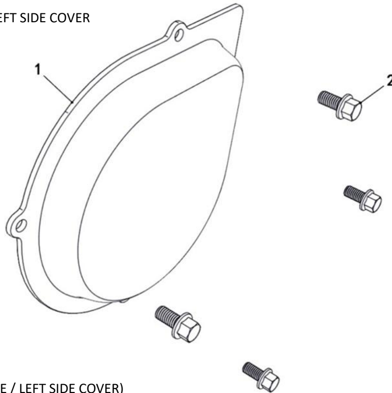
DELE TIL FIG 20 (COVER, VENSTRE SIDE / LEFT SIDE COVER)
