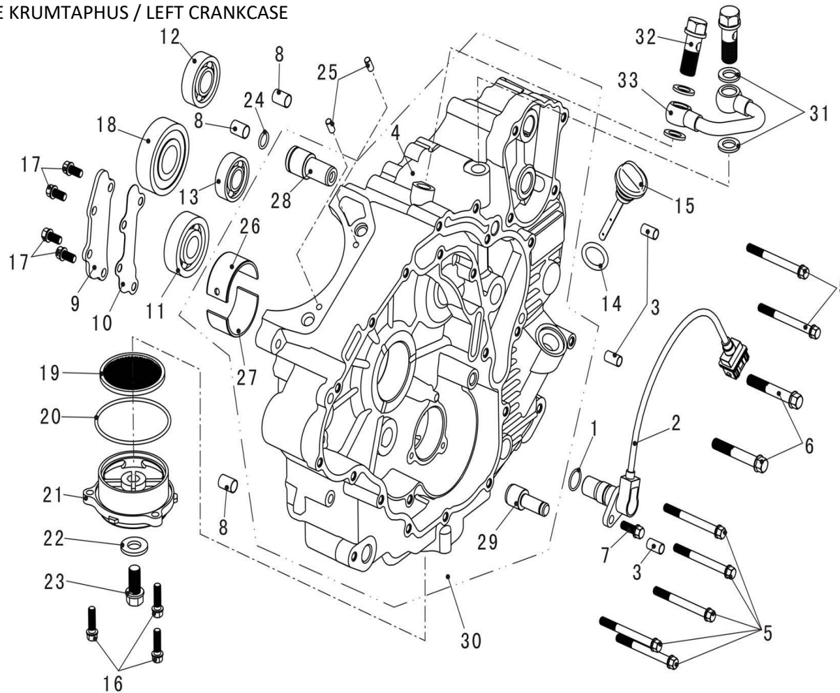
DELE TIL FIG 6 (VENSTRE KRUMTAPHUS / LEFT CRANKCASE)
