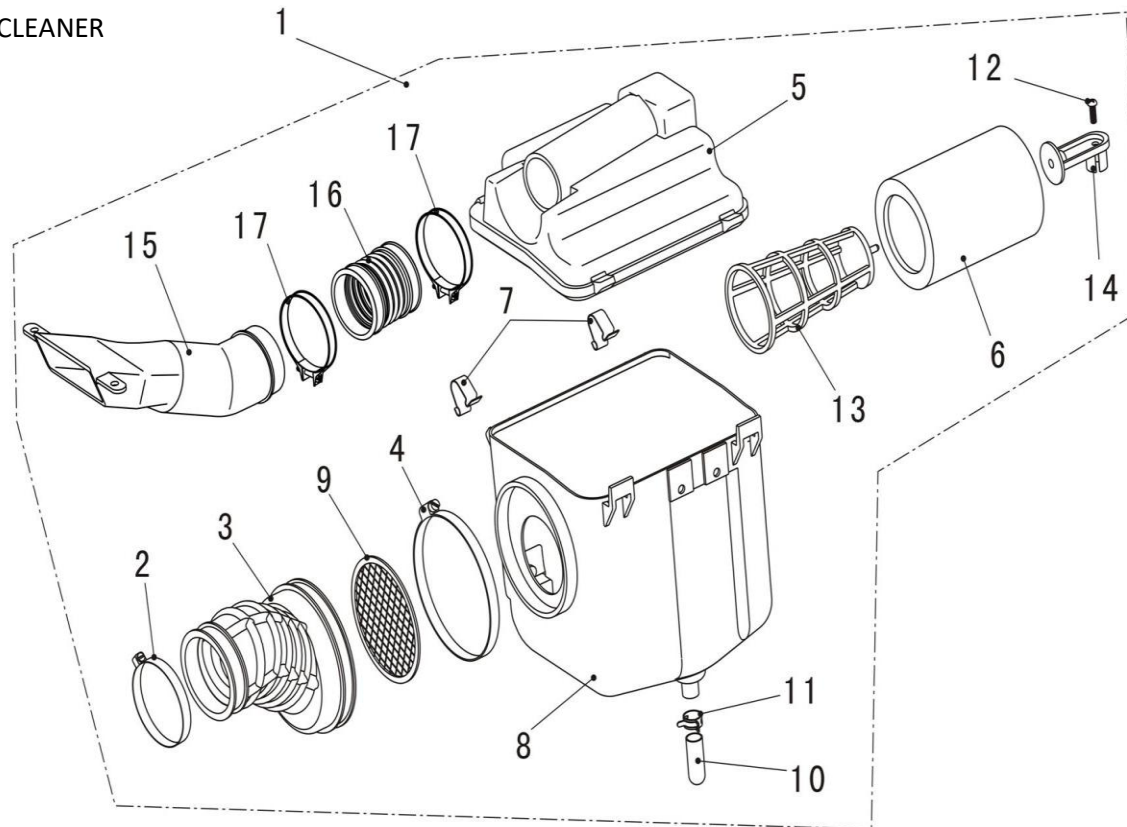
DELE TIL FIG 23 (LUFTFILTER / AIR CLEANER)
