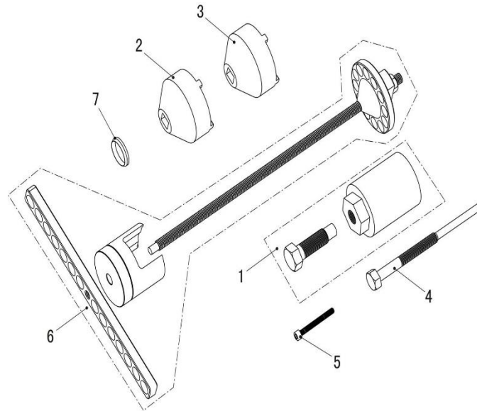
FIGUR 26 – SPECIALVÆRKTØJ / TOOLS
