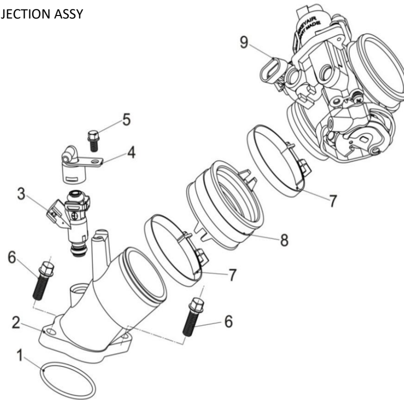
DELE TIL FIG 19 (GASSPJÆLDSSHUS / FUEL INJECTION ASSY)
