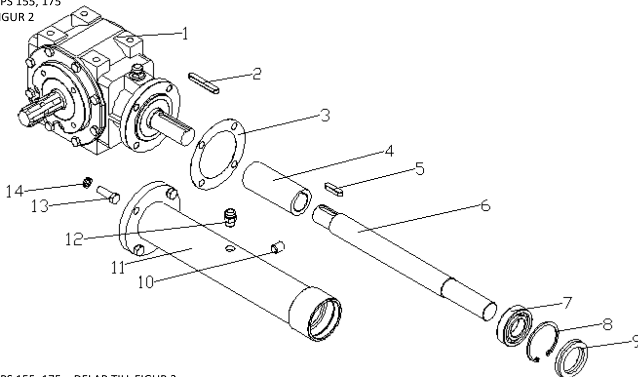
DPS 155, 175 – DELAR TILL FIGUR 2
