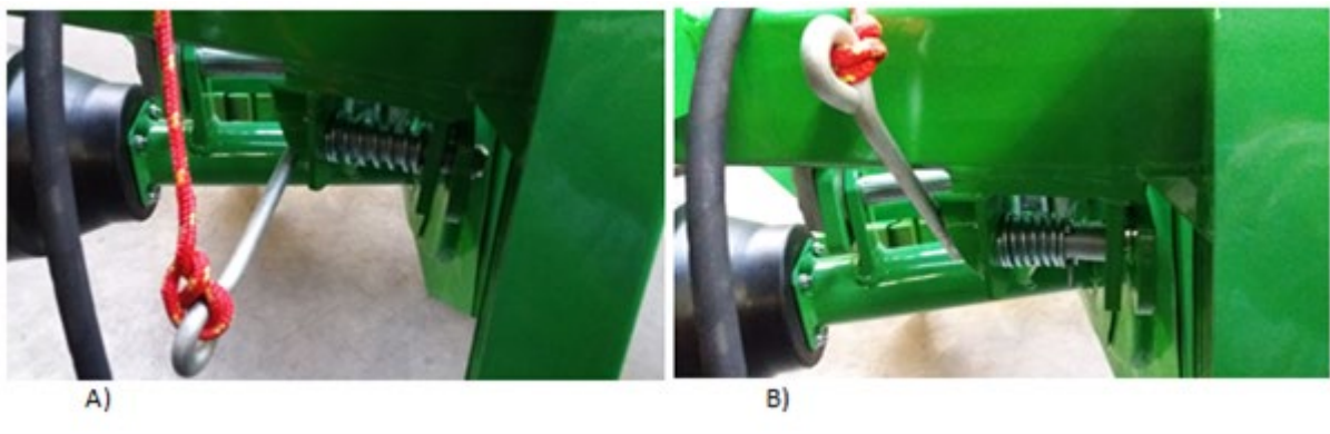
Upphängningens låssprint A= i gaffelbultens hål B=Urtaget ur hålet
