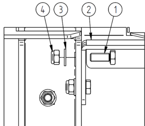
Detaillierte Abbildung der Bolzenelemente für Schritt 4
