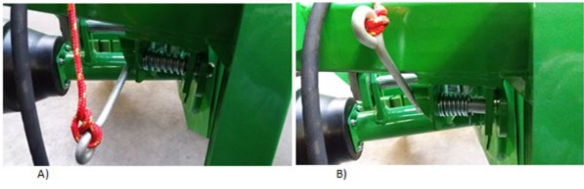
Sperrsplint des Hauptrahmens A= im Loch des Gabelbolzens B=aus dem Loch entfernt
