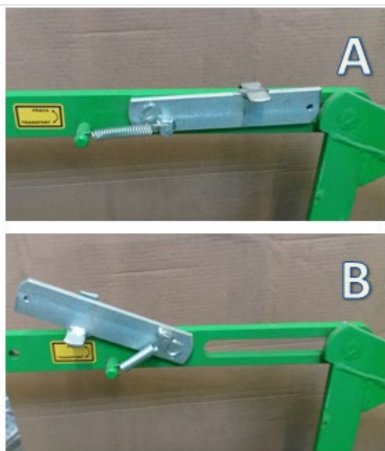
A = Transportposition B=Betriebsposition
