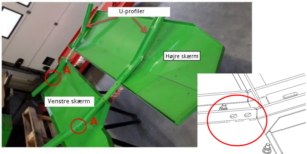
Detalje A
