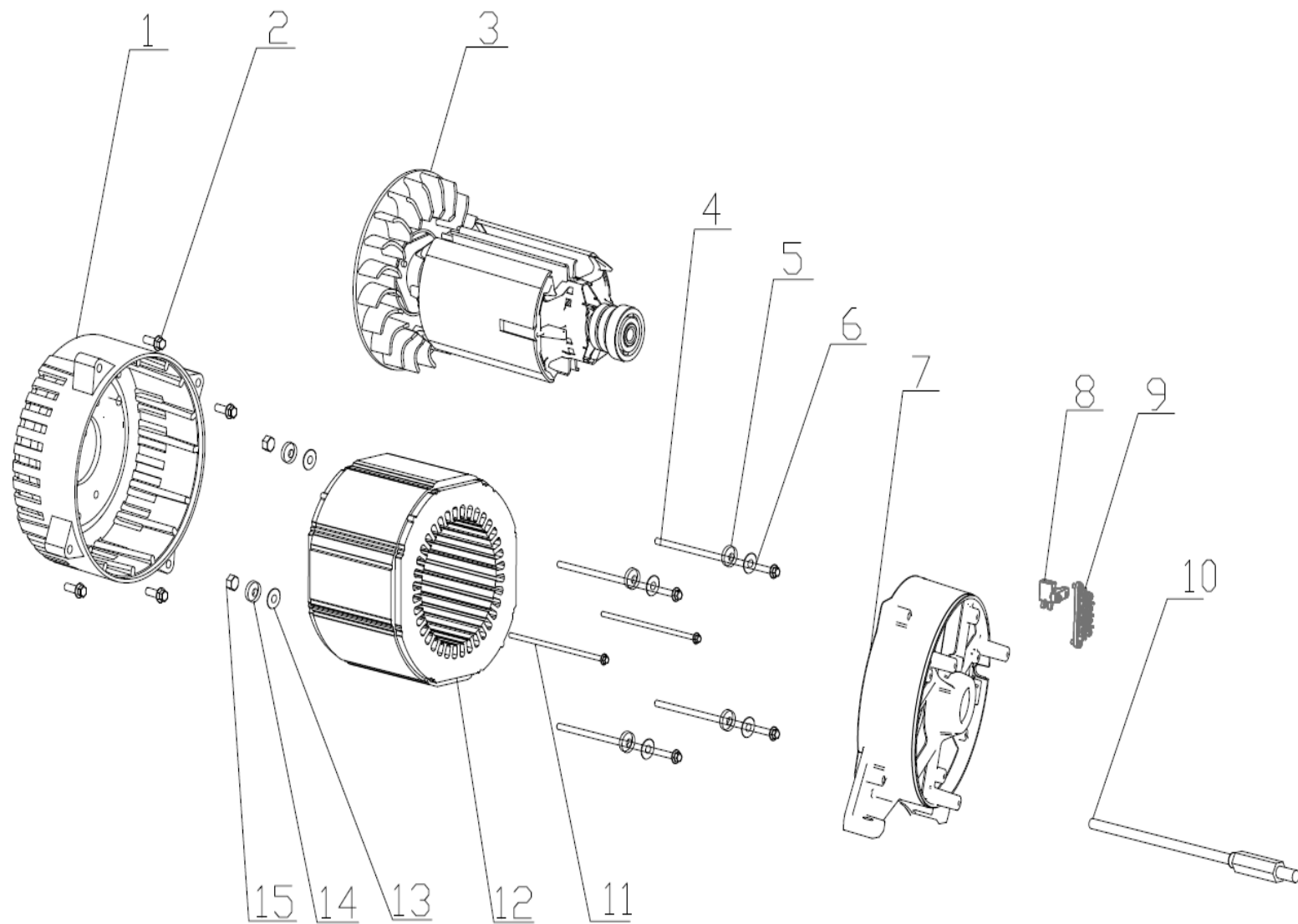
FIGUR 3 - MOTOR
