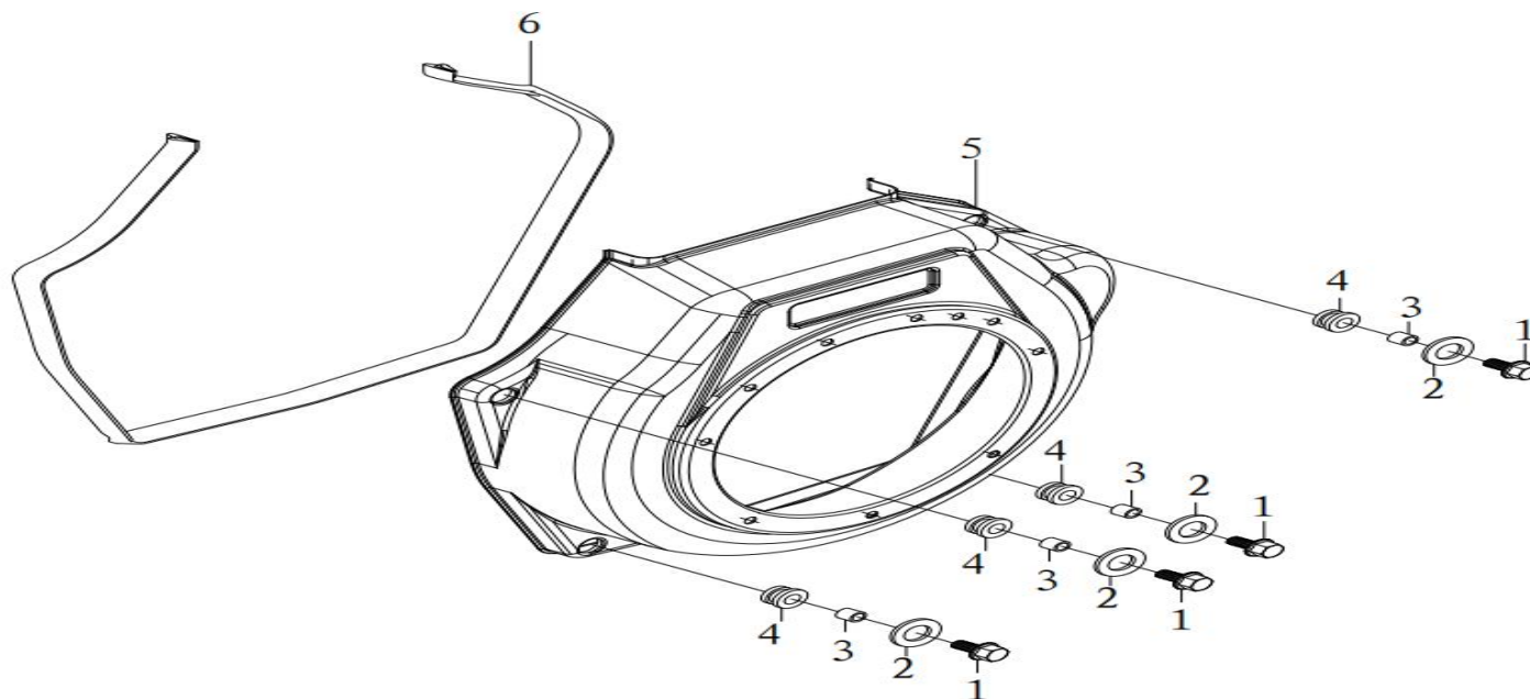
FIGUR E14 - VINDAVLEDARENHET
