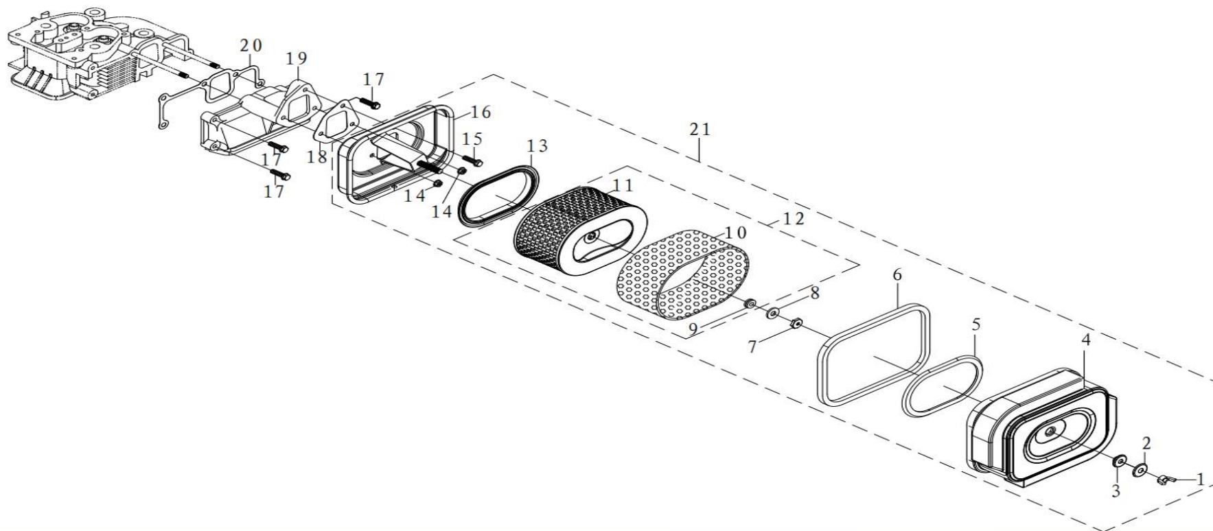
DELAR TILL FIG E15
