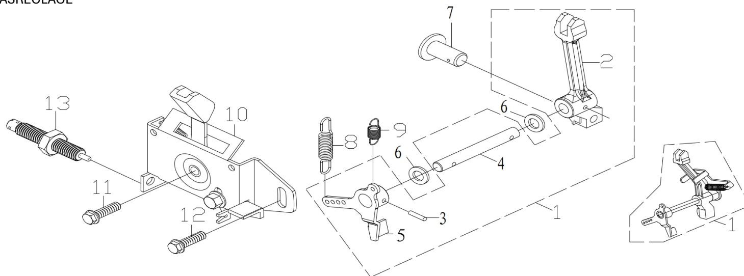
FIGUR E18 - GASREGLAGE
