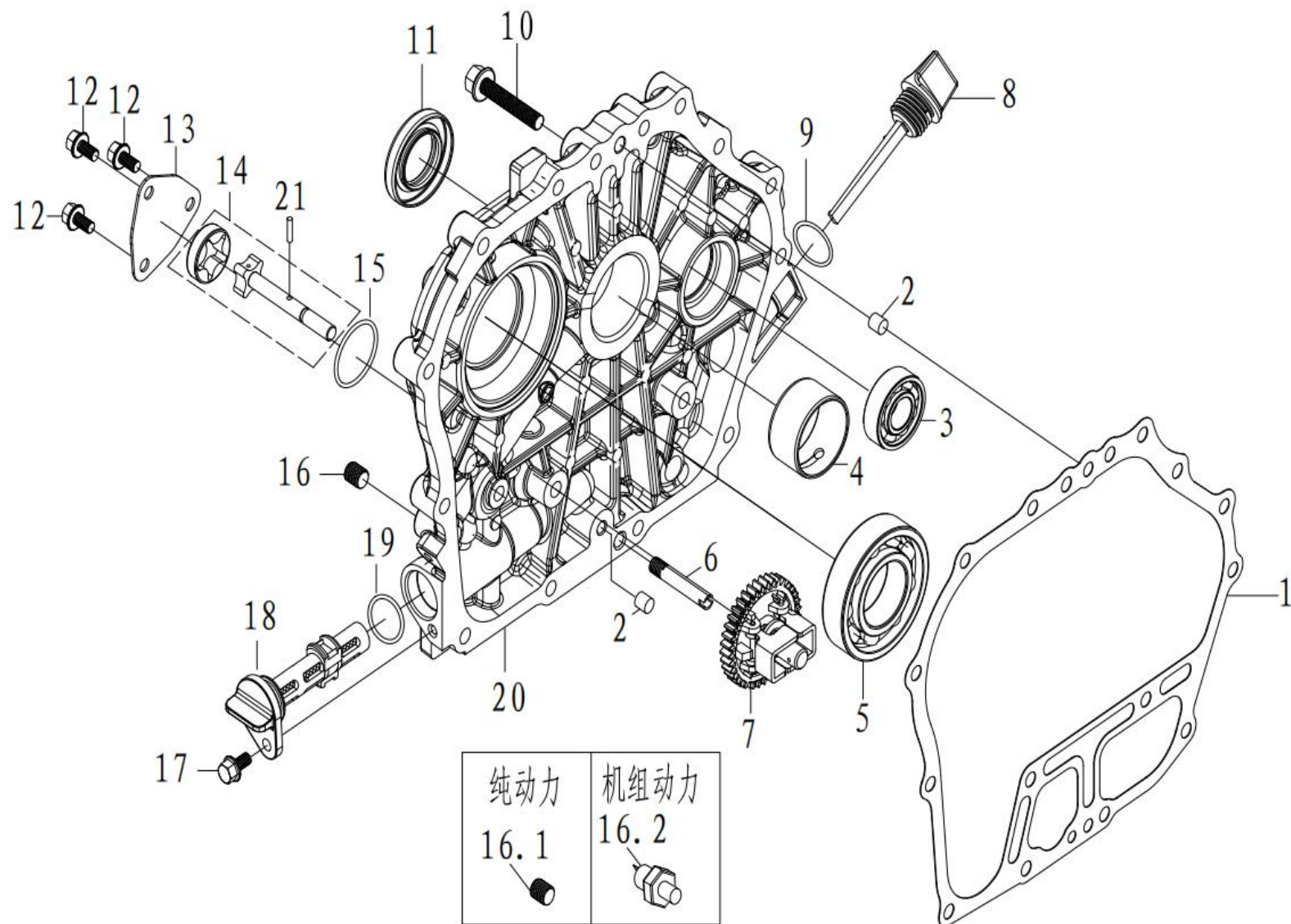
FIGUR E9 - VEVHUSLOCK
