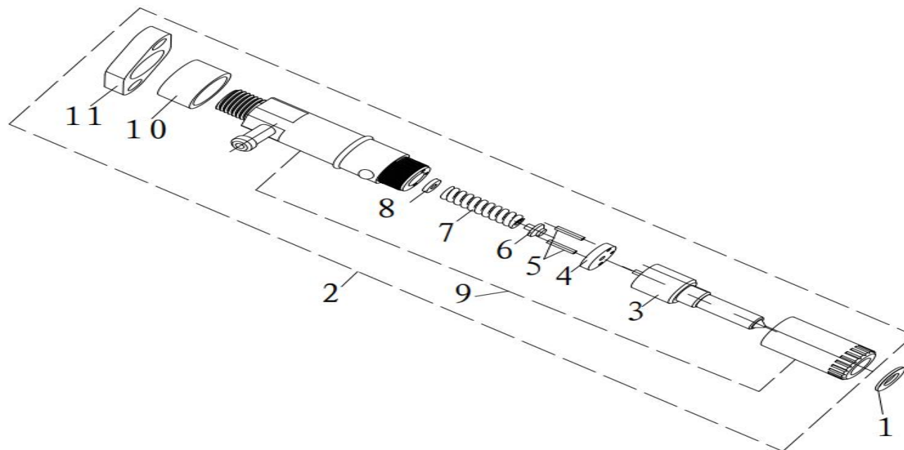
FIGUR E17 - BRÄNSLEINSPRUTNINGSENHET
