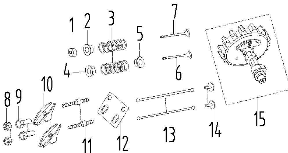
MOTOR FIGUR 5 – KNASTAKSEL / CAMSHAFT
