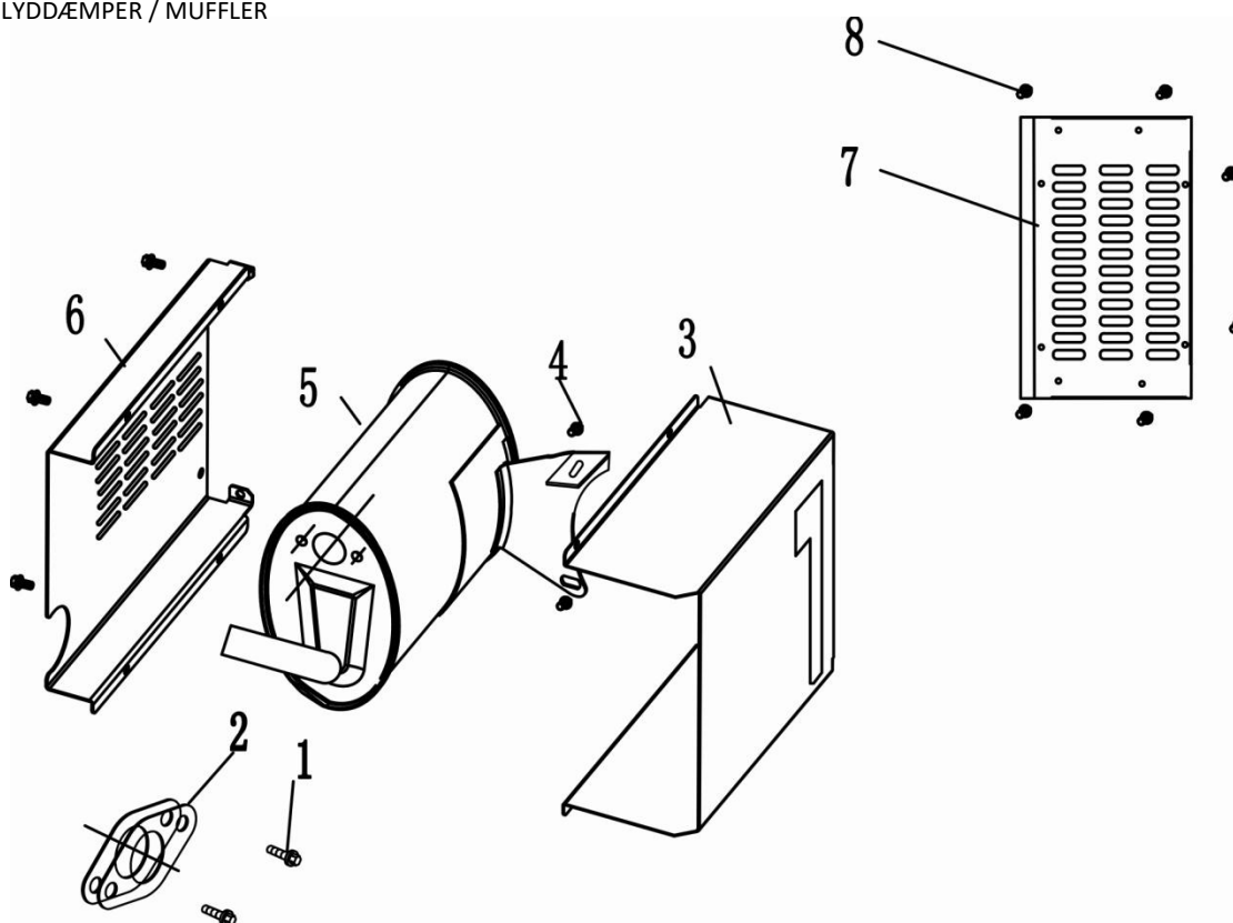
FIGUR 6 – LYDDÆMPER / MUFFLER
