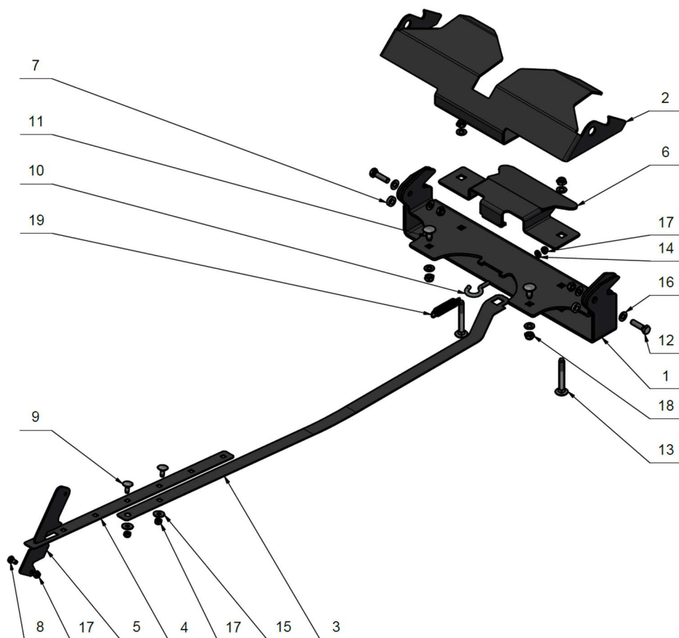
BILD. 17: Teileschema 4
