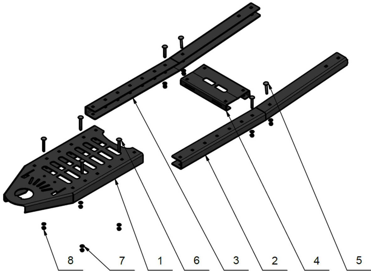
BILD. 16: Teileschema 3
