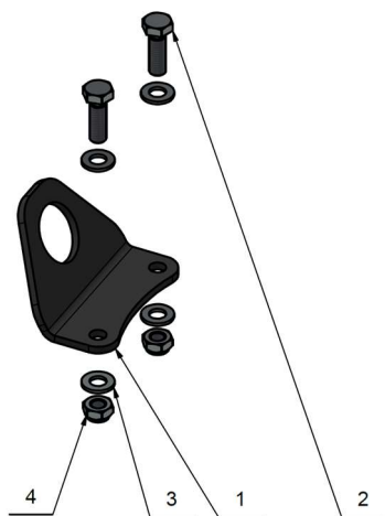
BILD. 18: Teileschema 5
