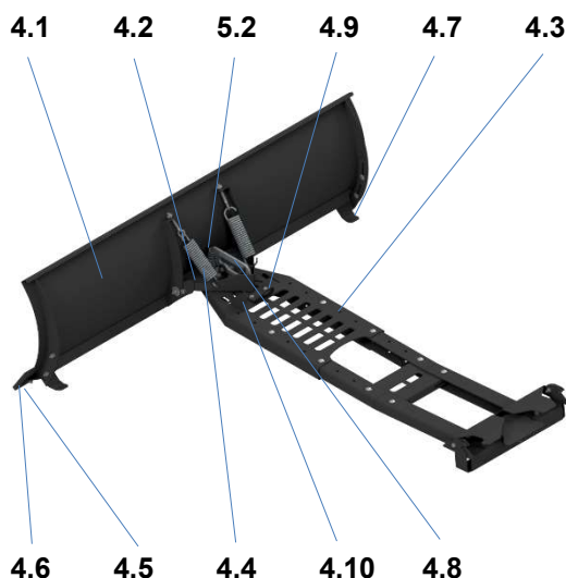
BILD. 4: Snowblade-Beschreibungsansicht A
