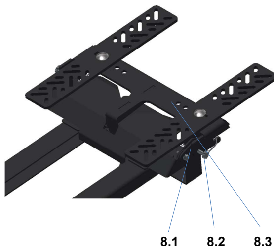
BILD. 8: Hinterer Teil des Hauptrahmens
