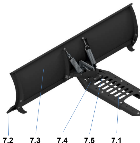
BILD. 7: Vorderer Teil des Hauptrahmens
