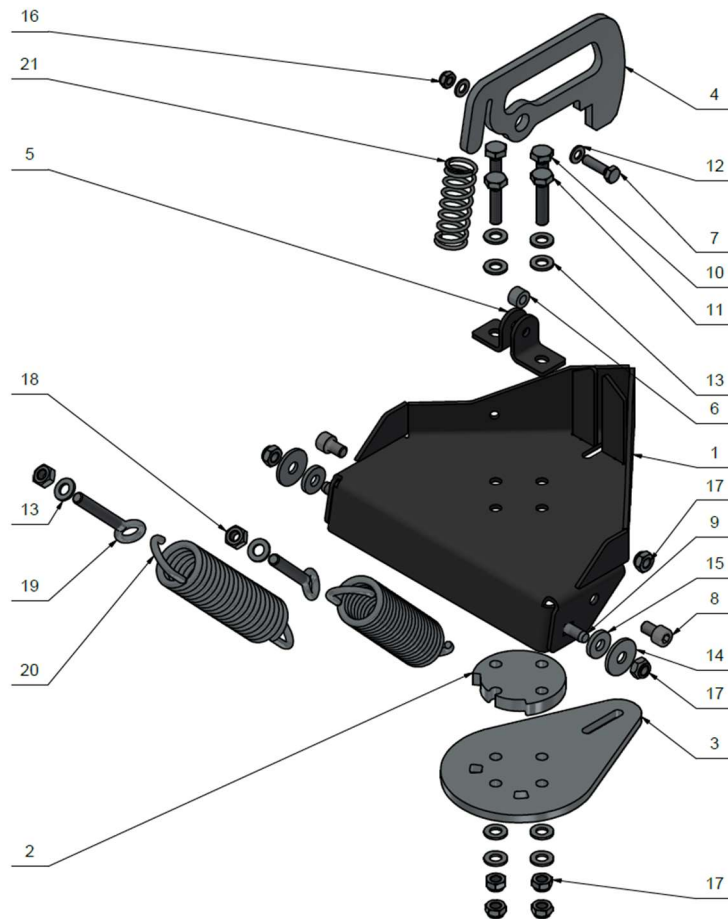
BILD. 15: Teileschema 2
