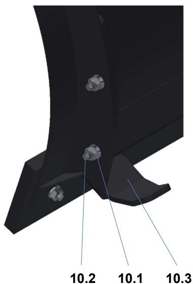
BILD. 10: Gleitschuheinstellung
