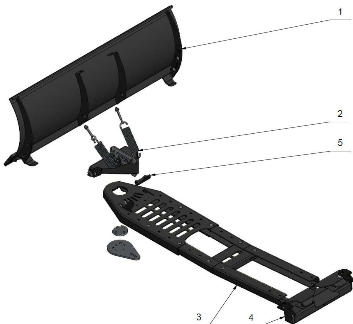
BILD. 13: Teileschema
