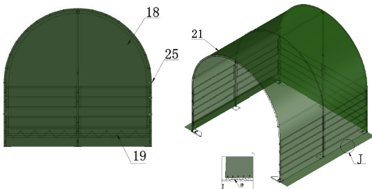
FIGUR 5 – endegavl og tag
