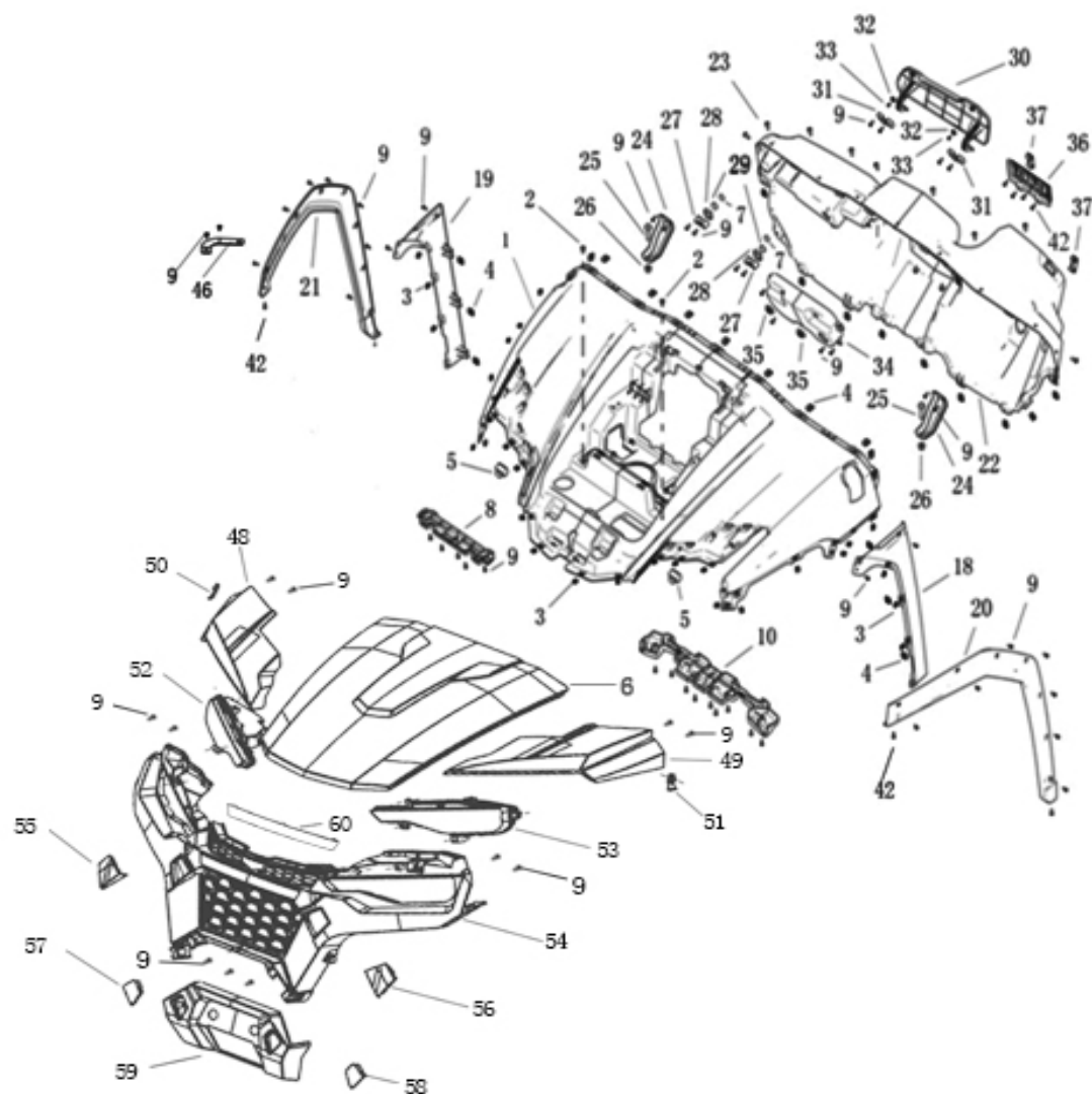
FIGUR 5 – FORSKÆRM &amp; HJELM / FRONT FENDER
