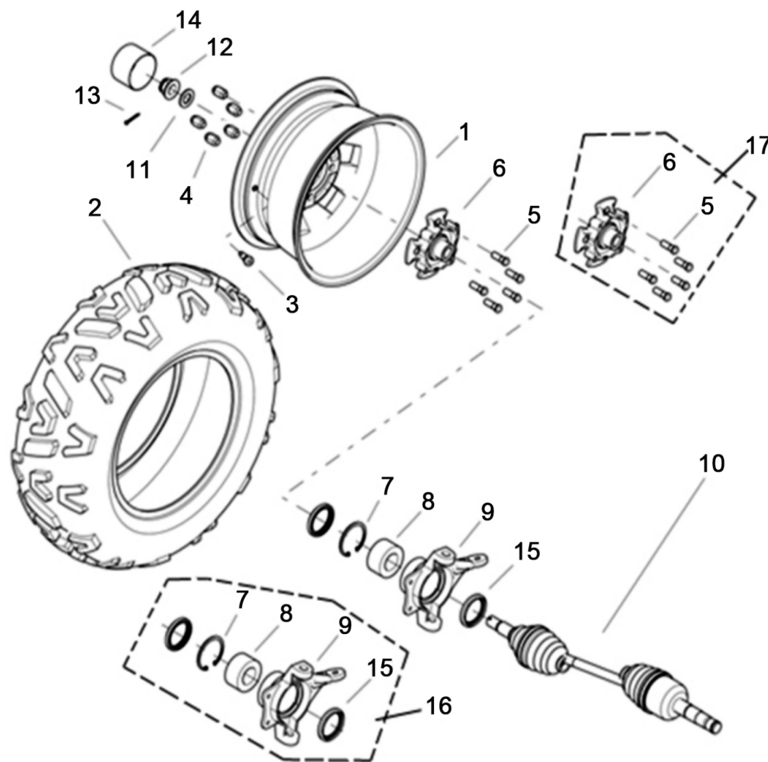
FIGUR 29 – HØJRE FORHJUL / FRONT WHEEL, RIGHT
