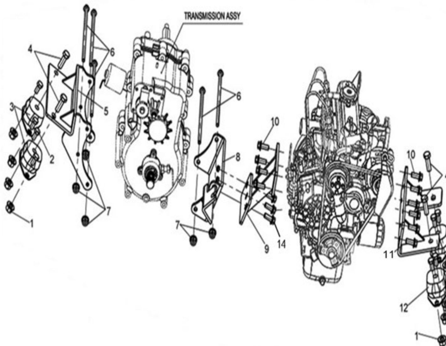
FIGUR 24 – MOTORPHÆNG & GEAR / ENGINE & TRANSMISSION
