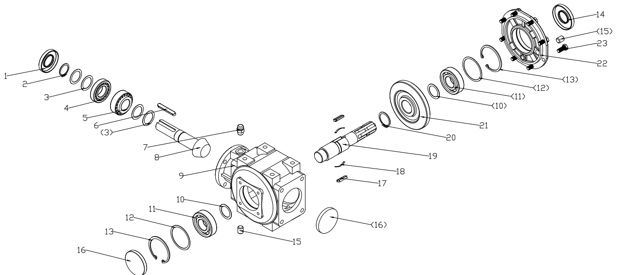
FIG. 3 VINKELVÄXELNS DELAR
