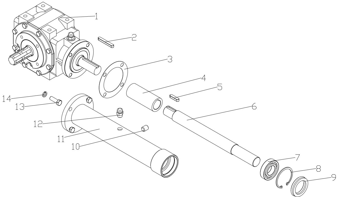
ABB. 2 GETRIEBE
