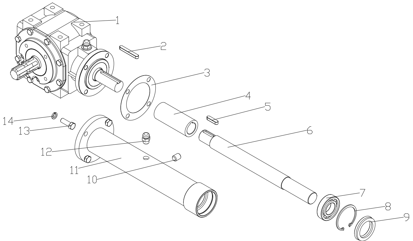
FIG. 3 – GEARKASSEDELE
