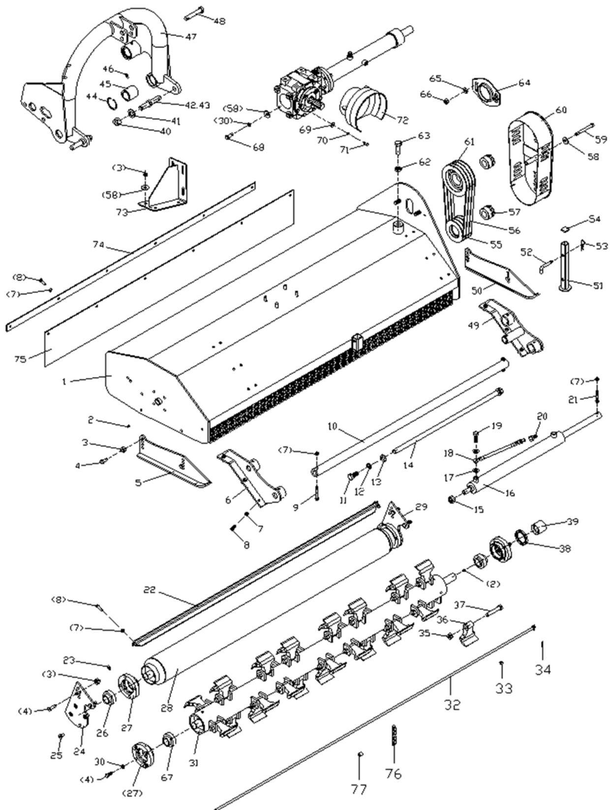
FIG. 1 HUVUDMASKIN
