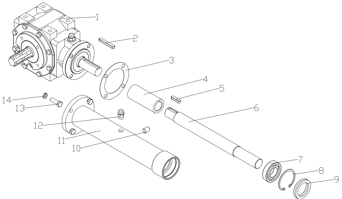
FIG. 3 VINKELVÄXELNS DELAR
