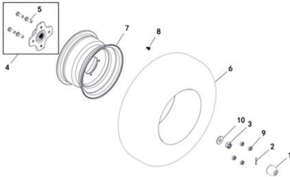
DELE TIL FIG 9 (BAGHJUL / REAR WHEEL)
