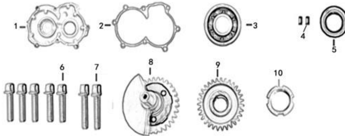
DELE TIL FIG E7 (KRUMTAP II / CRANKCASE II)
