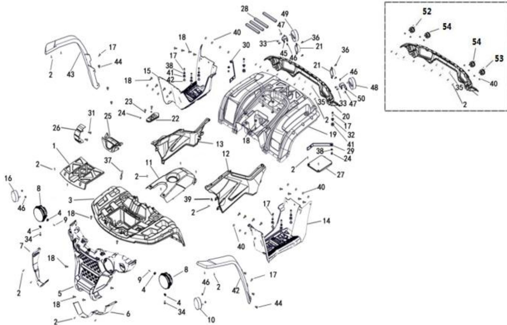
FIGUR 5 – SKÆRMDELE / FENDERPARTS
