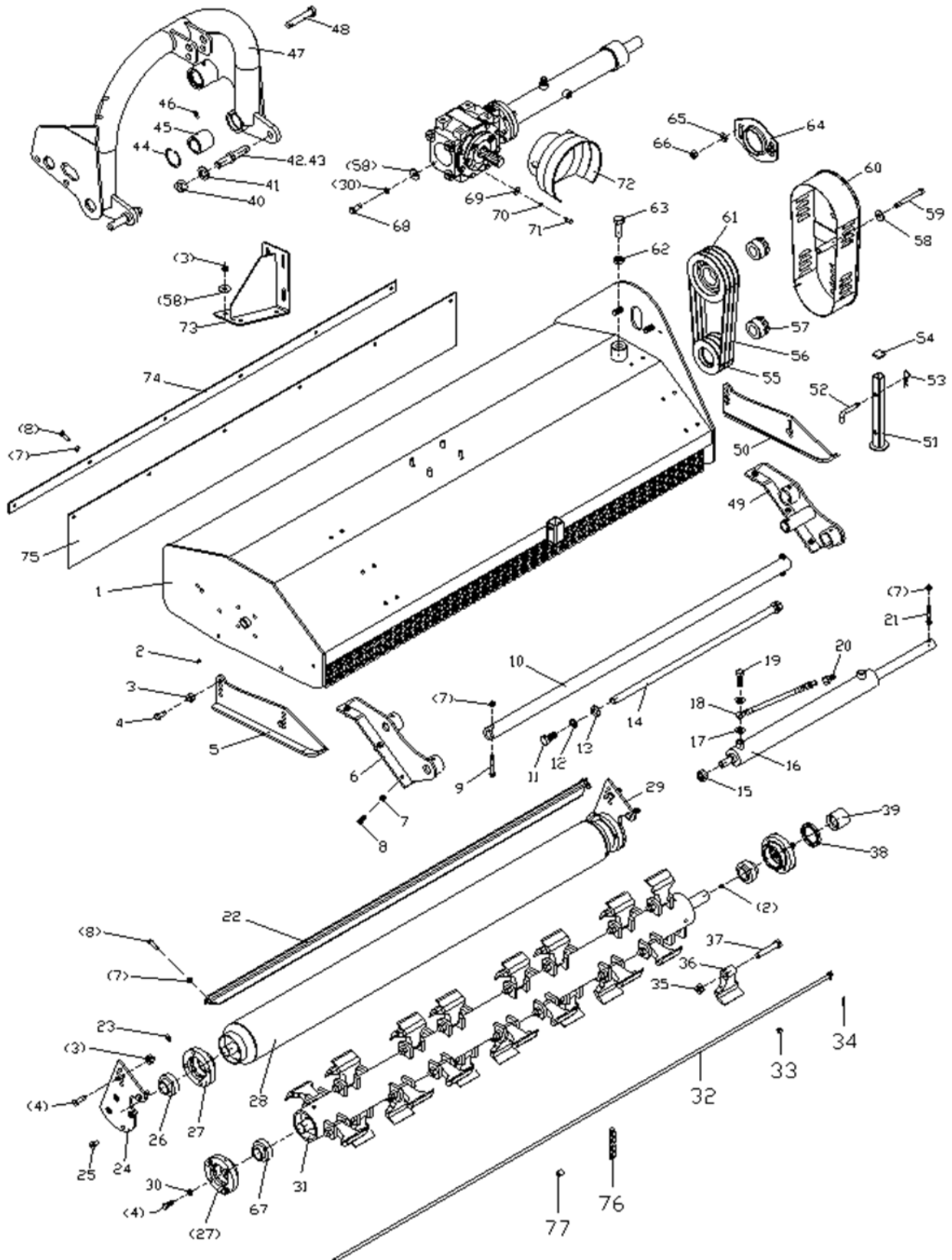
FIG. 1 HUVUDMASKIN
