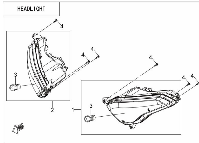
FIGUR 8 – FORLYGTER
