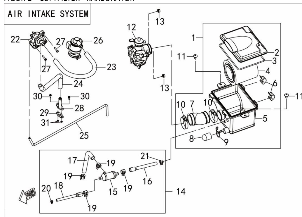
FIGUR 2 – LUFTFILTER - KARBURATOR
