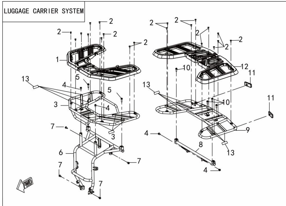
FIGUR 18 – BAGAGEBÆRER
