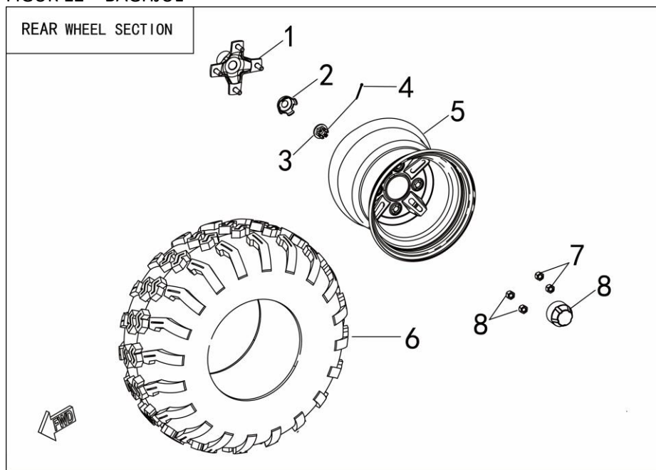
FIGUR 12 – BAGHJUL
