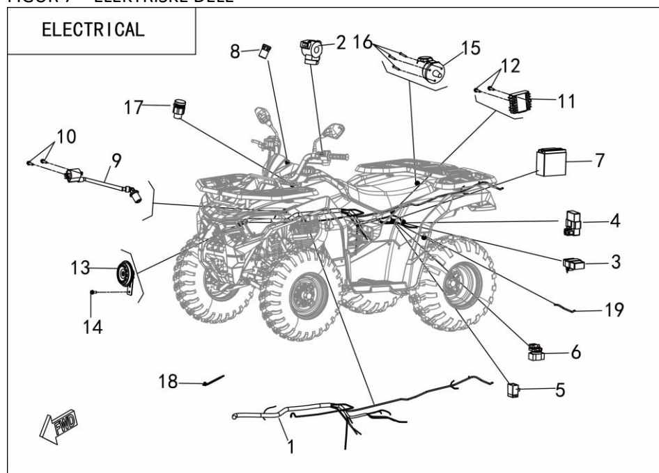
FIGUR 7 – ELEKTRISKE DELE
