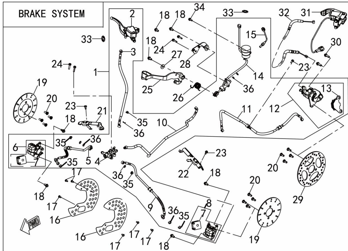
FIGUR 10 – BREMSESYSTEM
