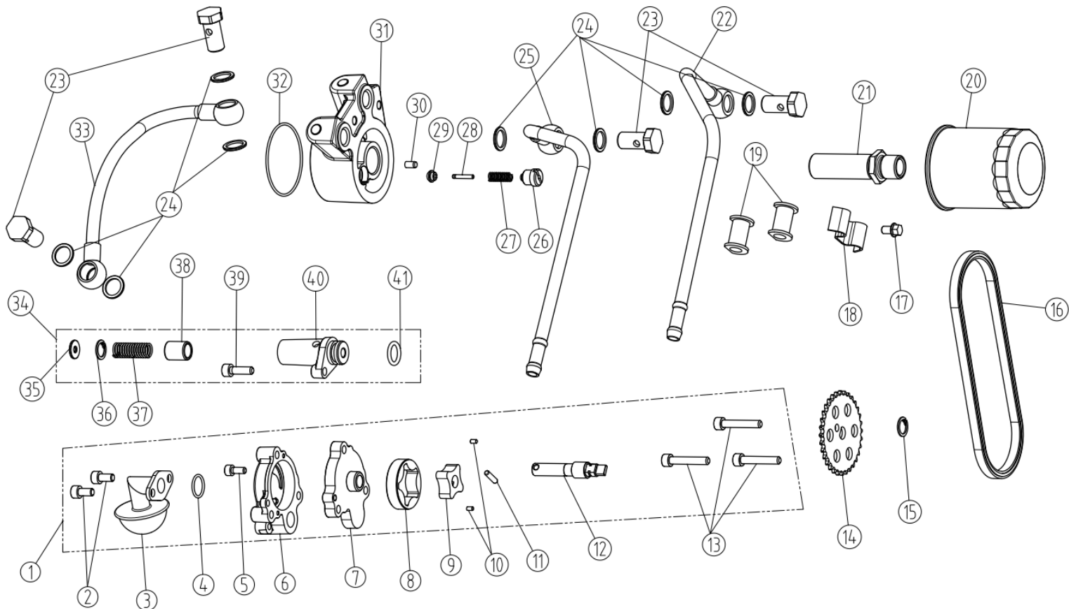
MOTOR FIGUR E9 – OLIESMØRING
