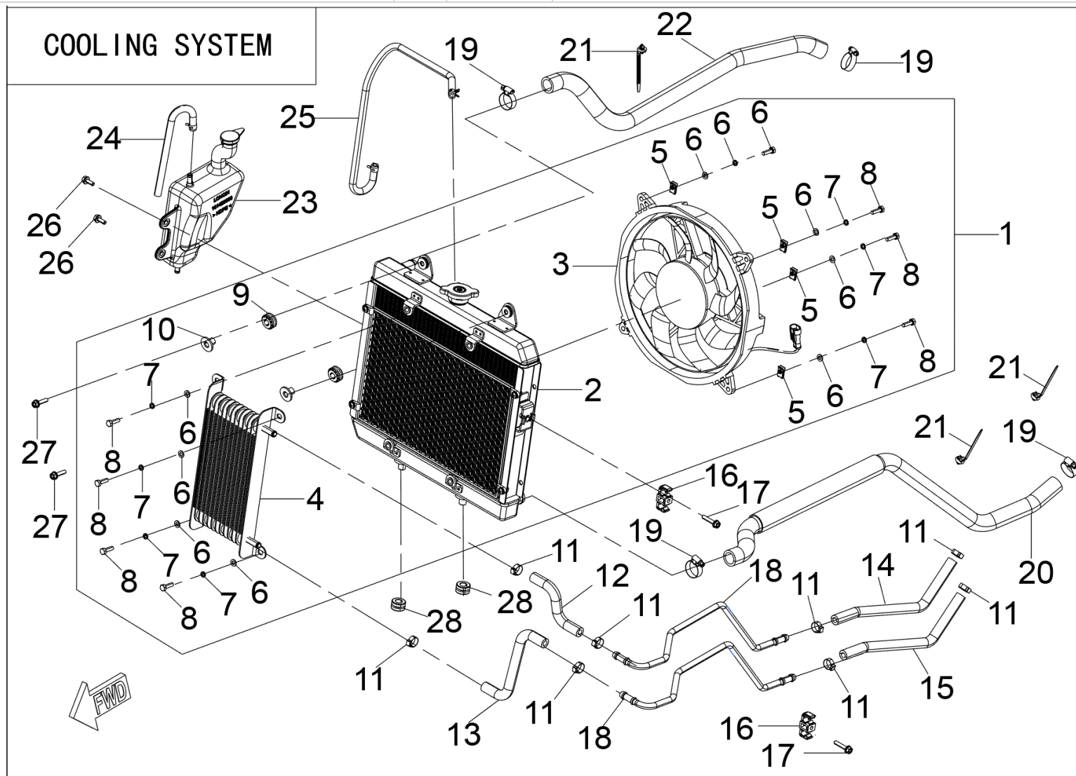
FIGUR 1 – KØLESYSTEM
