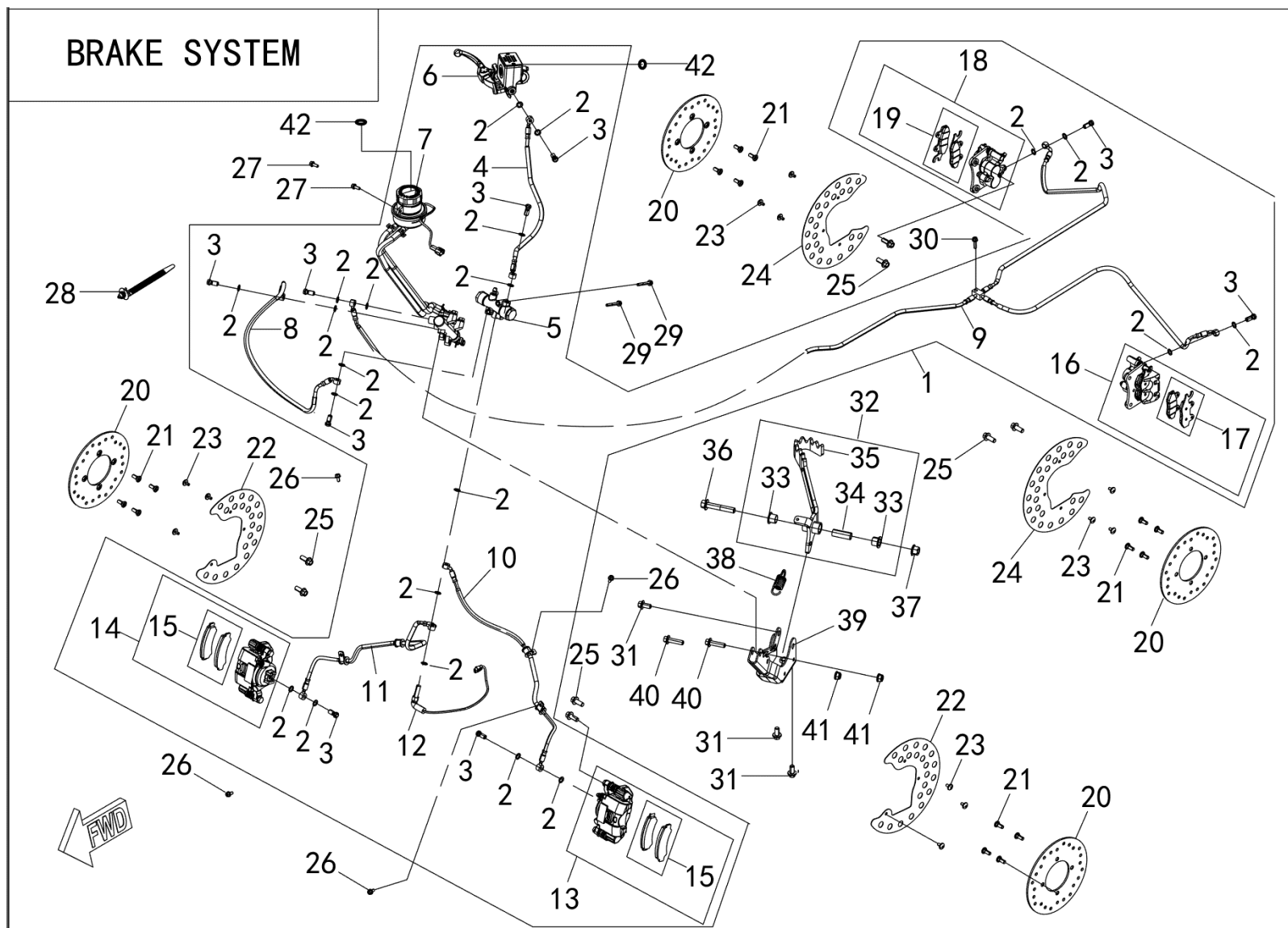
FIGUR 13 – BREMSESYSYSTEM
