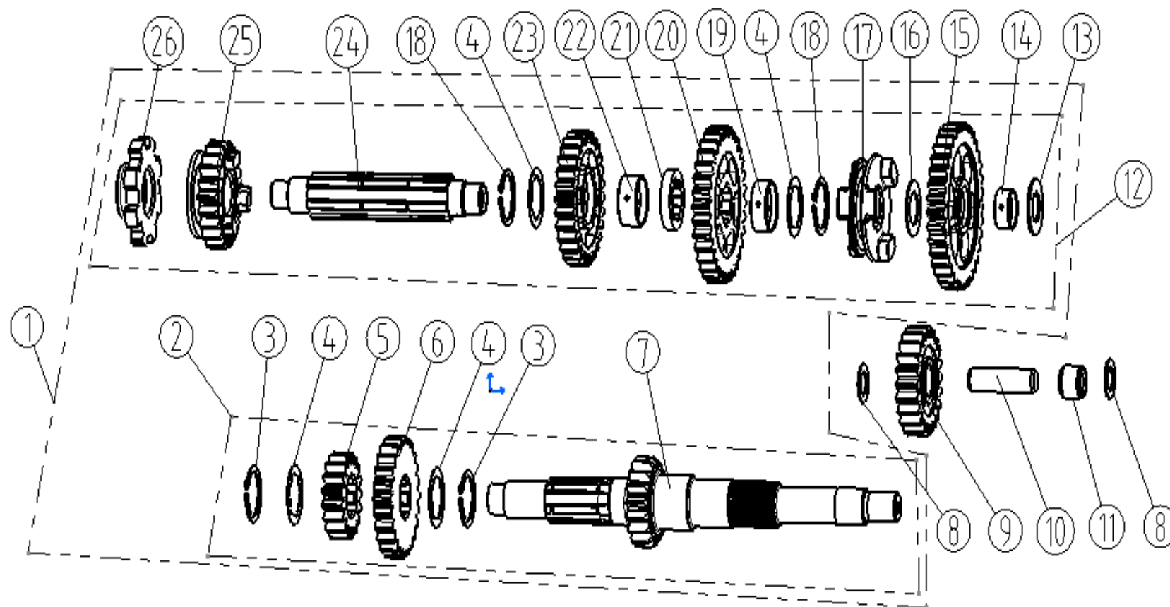
MOTOR FIGUR E12 – HOVEDAKSEL & UDGANGSAKSEL
