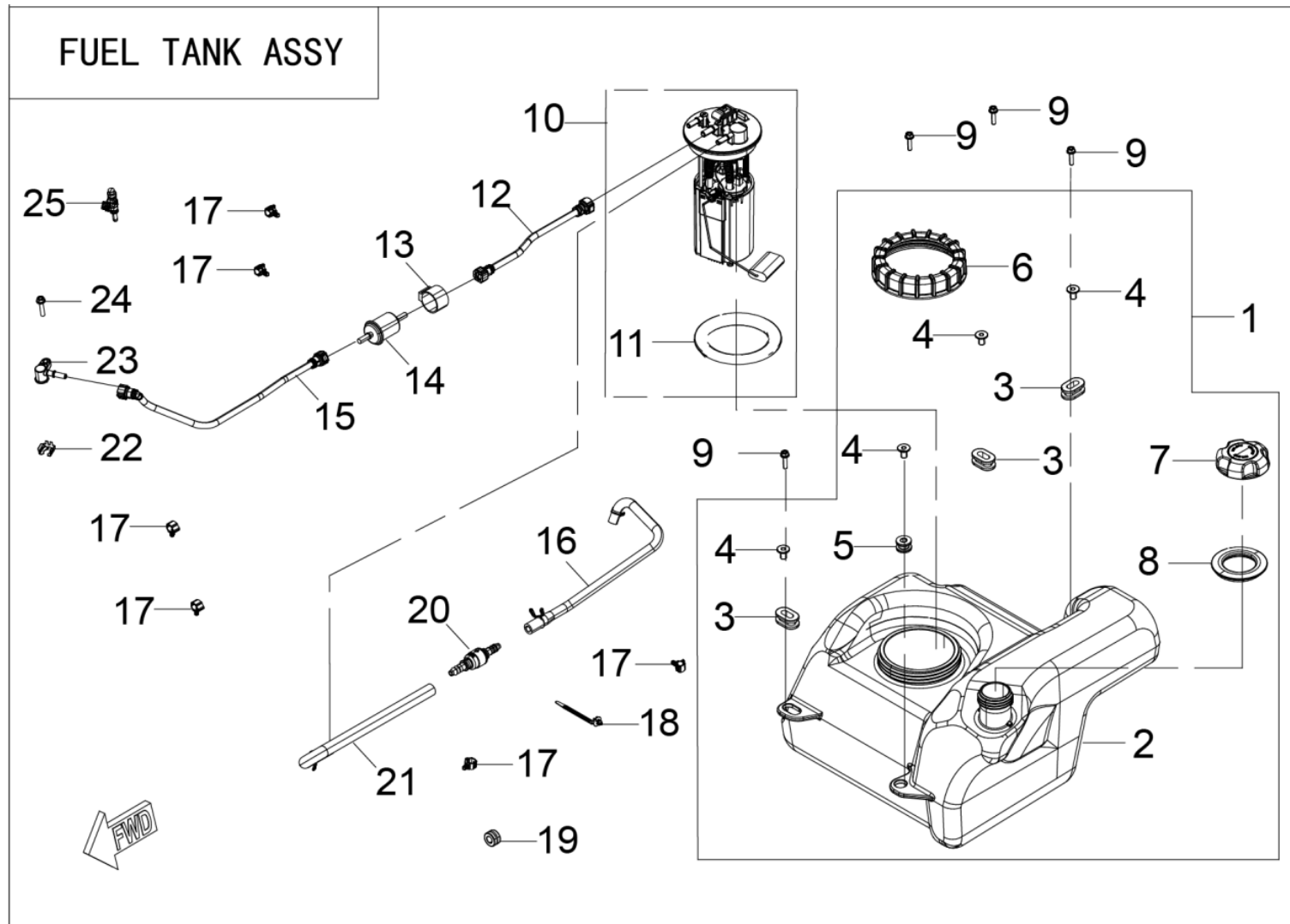
FIGUR 2 – BRÆNDSTOFTANK
