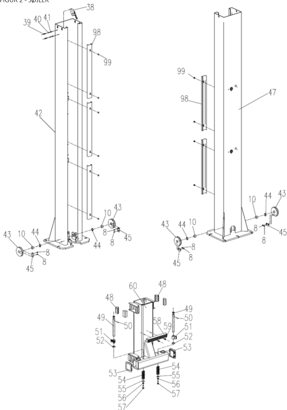
FIGUR 2 - SØJLER
